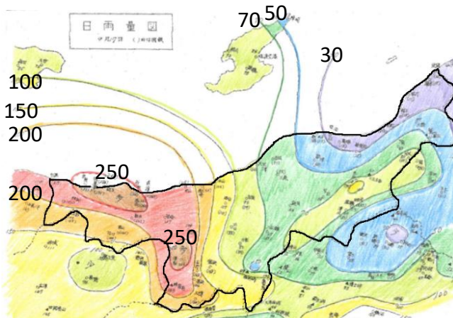
積算降水量（9月17日10時～9月18日09時）単位：ミリ
