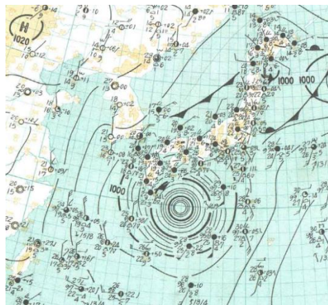
地上天気図（昭和40年9月17日09時）
