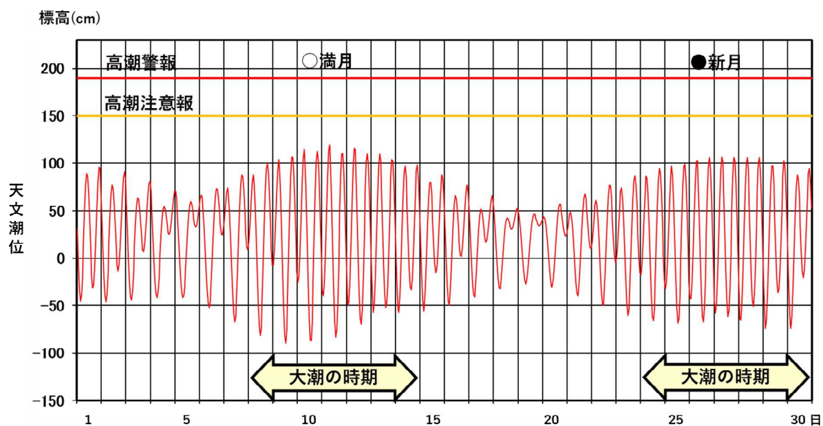
図3 奄美における2022年9月（1時間ごとの）の天文潮位
