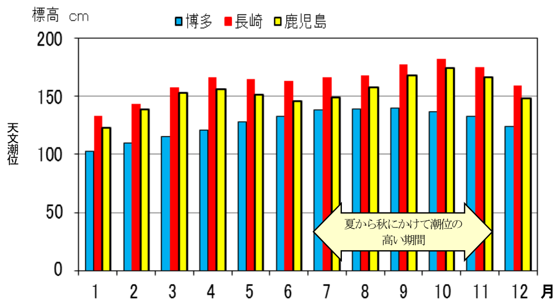
図2 博多・長崎・鹿児島における2021年の各月最高の天文潮位
