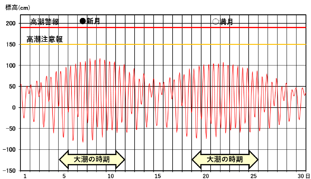
図3 奄美における2021年9月（1時間ごとの）の天文潮位
