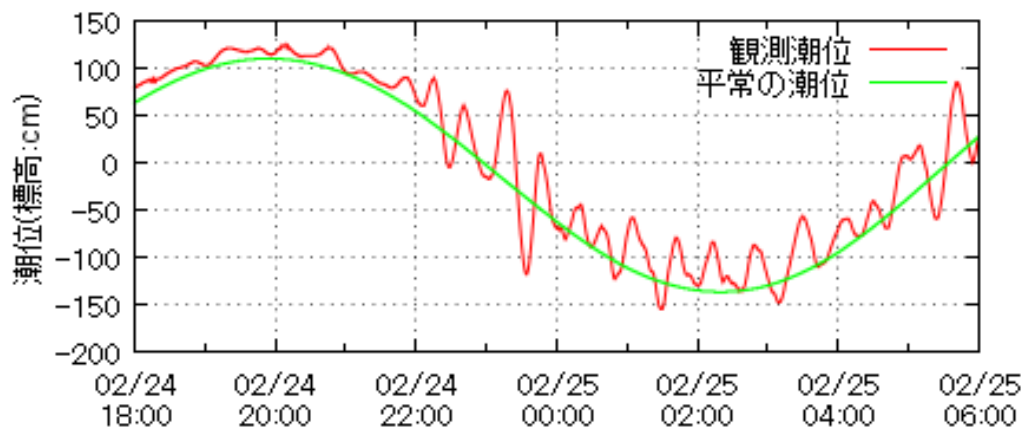
２００９年２月２４～２５日に長崎で起こった副振動
