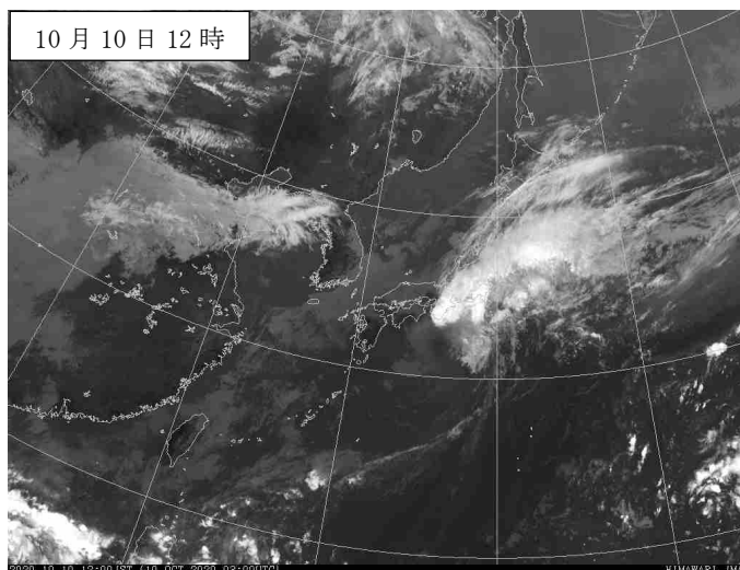
10月10日12時の地上天気図（左）と気象衛星赤外画像（右）
