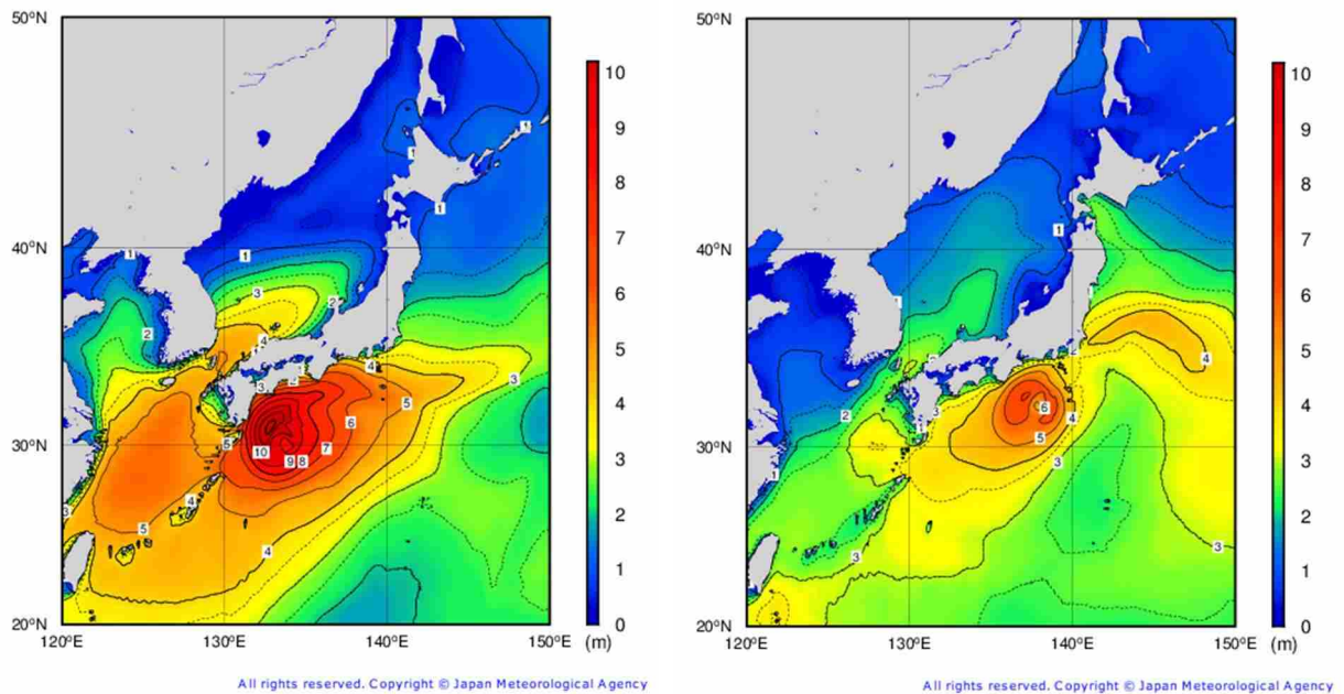
沿岸波浪実況図（左図：10月9日09時 右図：10月10日21時）
