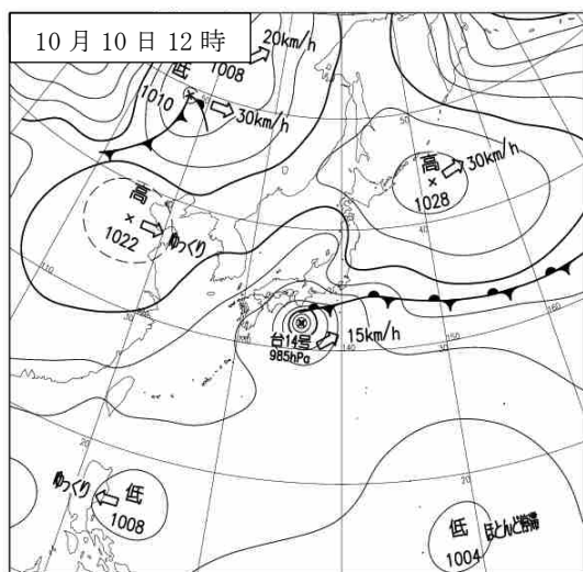
10月10日12時の地上天気図（左）と気象衛星赤外画像（右）
