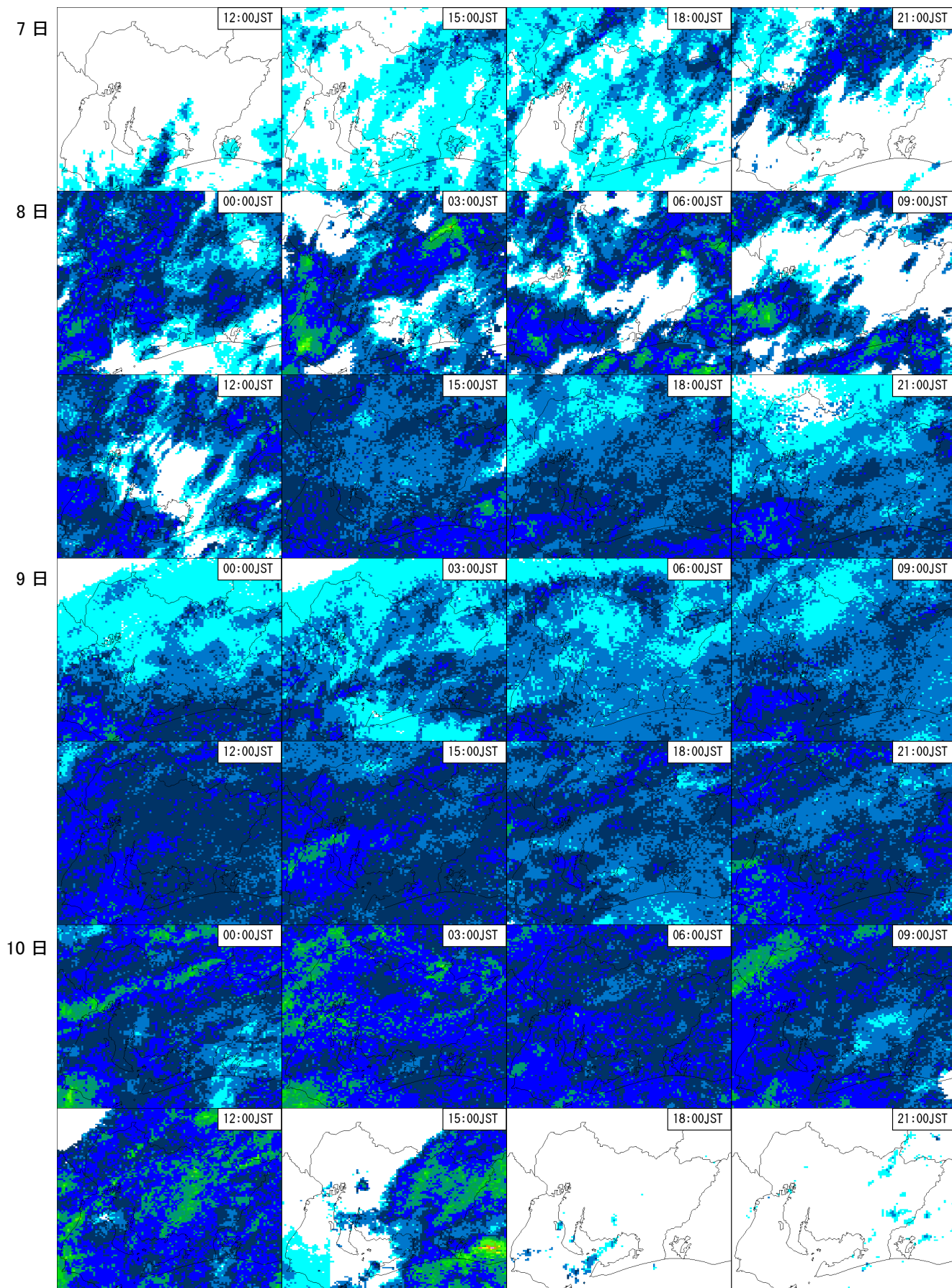
レーダーエコー合成図(10月7日12時00分～10日21時00分、3時間毎)
