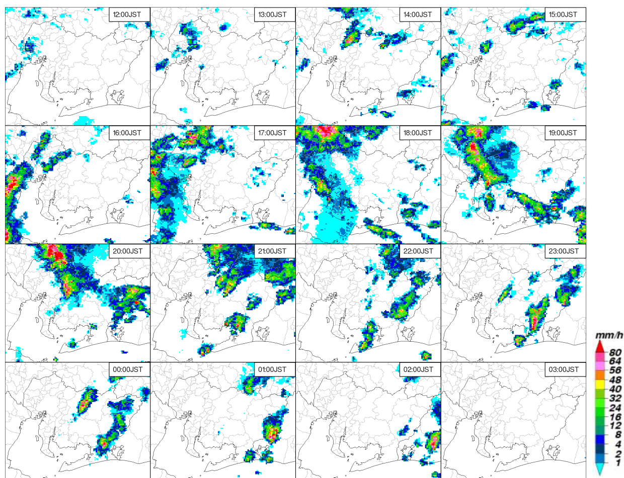
レーダーエコー合成図（8月25日12時～26日03時、1時間毎）
