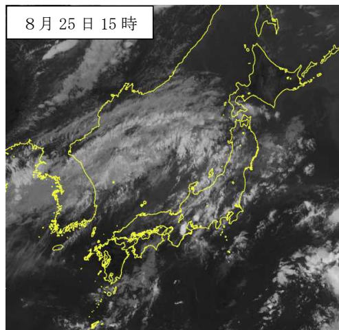
8月25日15時の地上天気図（左）と気象衛星赤外画像（右）
