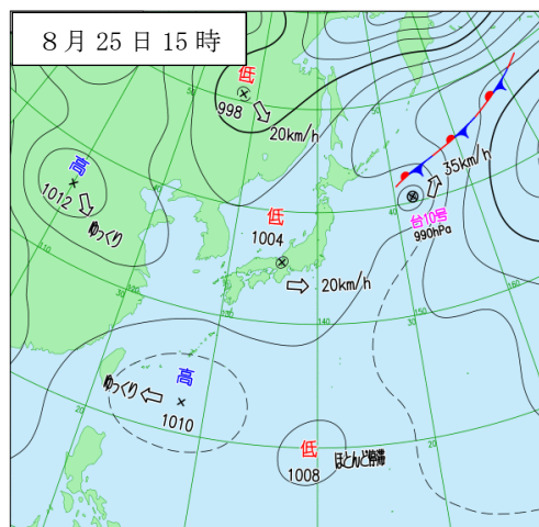
8月25日15時の地上天気図（左）と気象衛星赤外画像（右）
