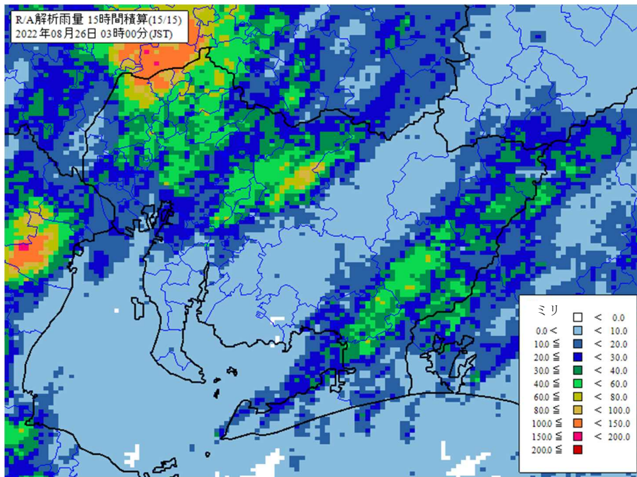
解析雨量積算図（8月25日12時～26日03時）
