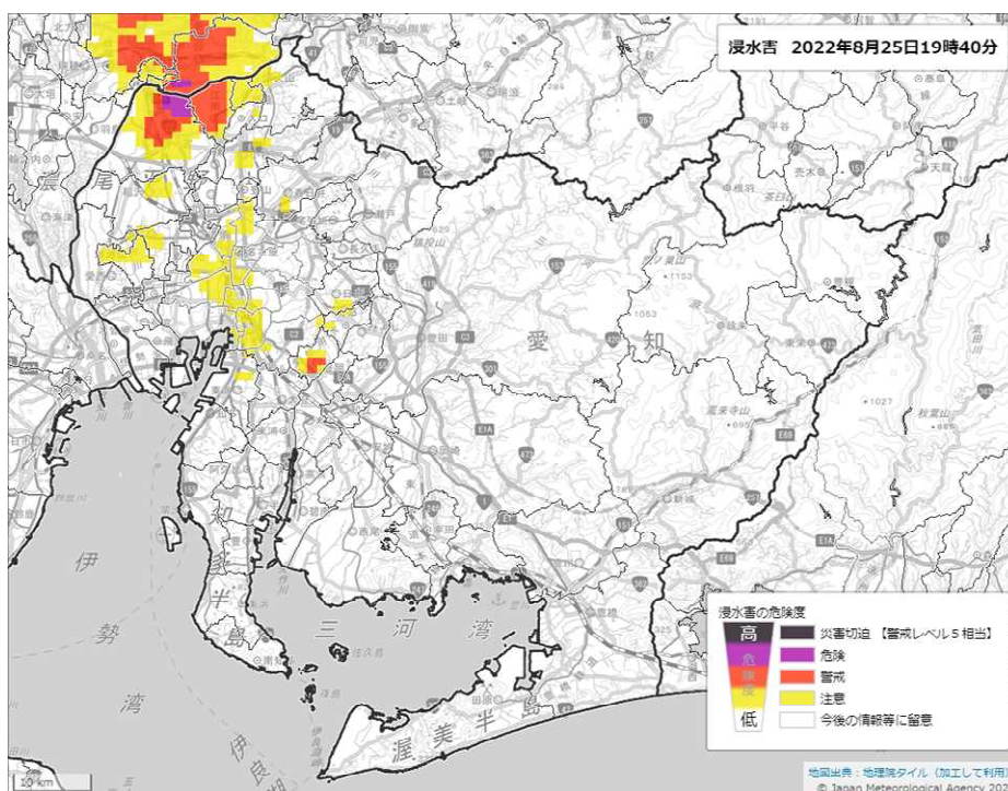
浸水キキクル（8月25日19時40分）
