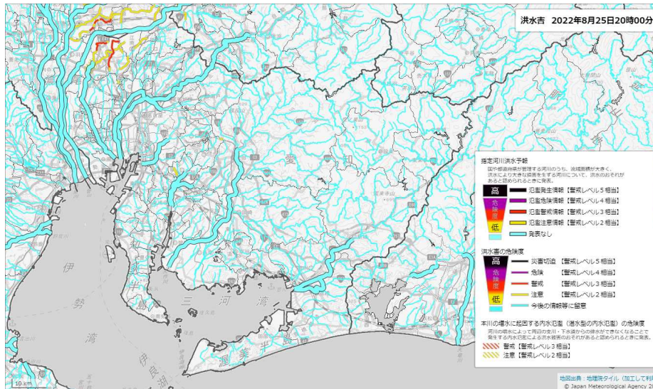
洪水キキクル（8月25日20時00分）
