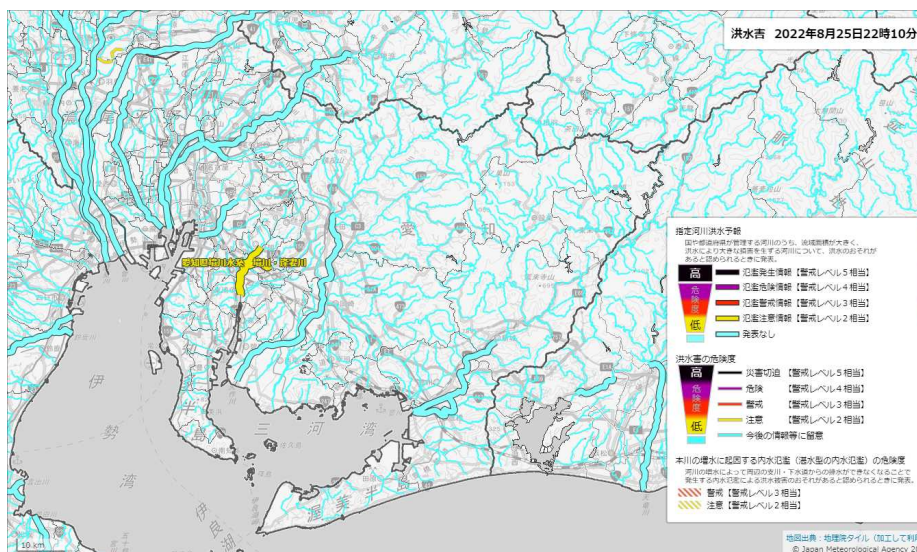
洪水キキクル（8月25日22時10分）
