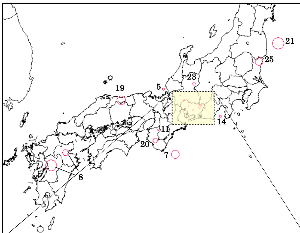
2016 年月毎の地震の概況に掲げた震央分布図
