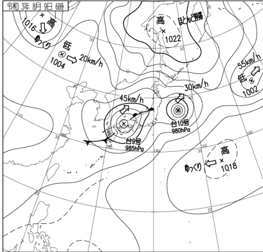
8月9日06時の地上天気図（左）と気象衛星赤外画像（右）
