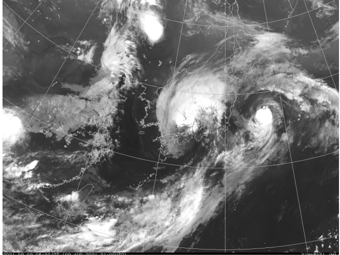
8月9日06時の地上天気図（左）と気象衛星赤外画像（右）
