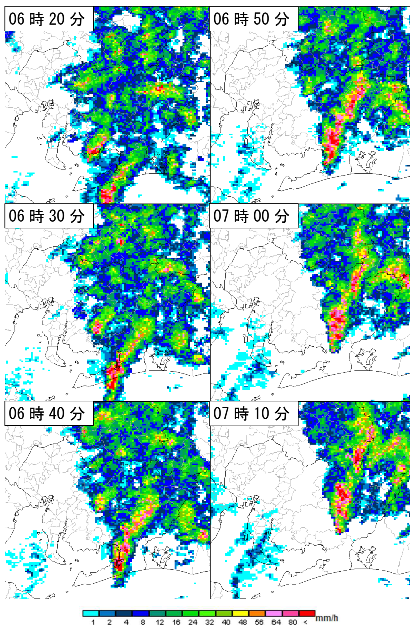
8月9日06時20分から10分毎のレーダー画像
