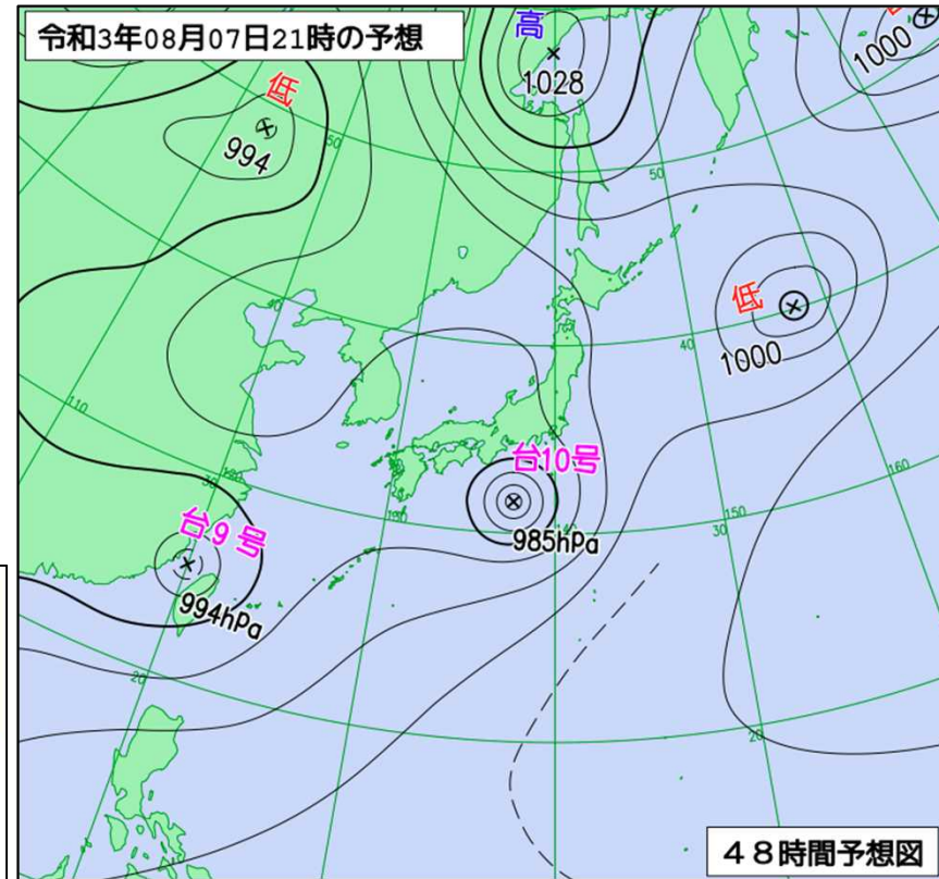
地上予想天気図 (8月7日21時の予想)
