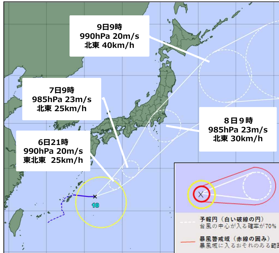
台風進路予想図 (8月6日9時の予想)
