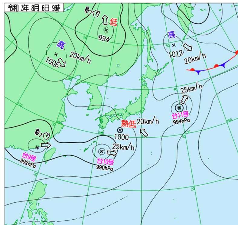
8月6日9時の気象衛星赤外画像（左）と9時の地上天気図（右）
