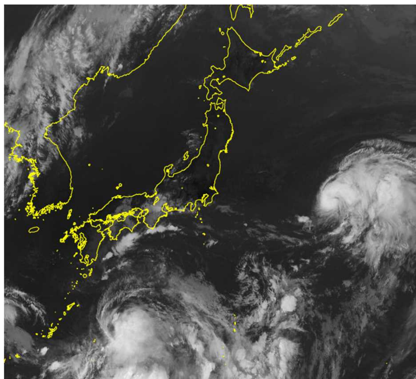
8月6日9時の気象衛星赤外画像（左）と9時の地上天気図（右）
