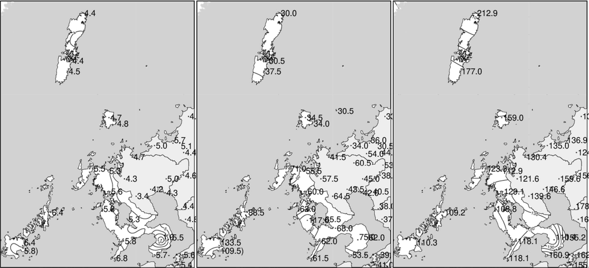
2025年2月気温観測値（℃）メッシュ平年値補正
