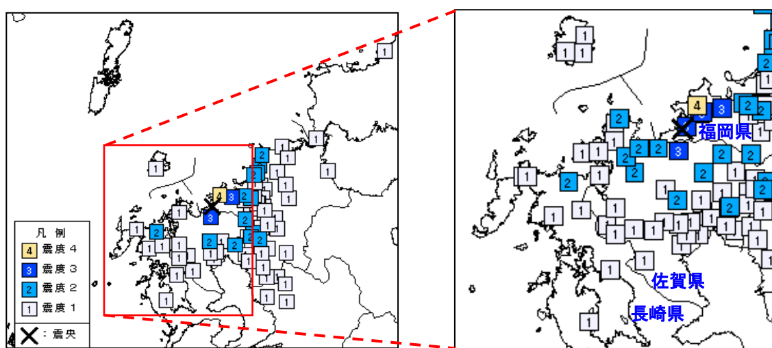
8月17日06時37分 M4.2 図8 震度分布図（左：市区町村別 右：観測点別）
