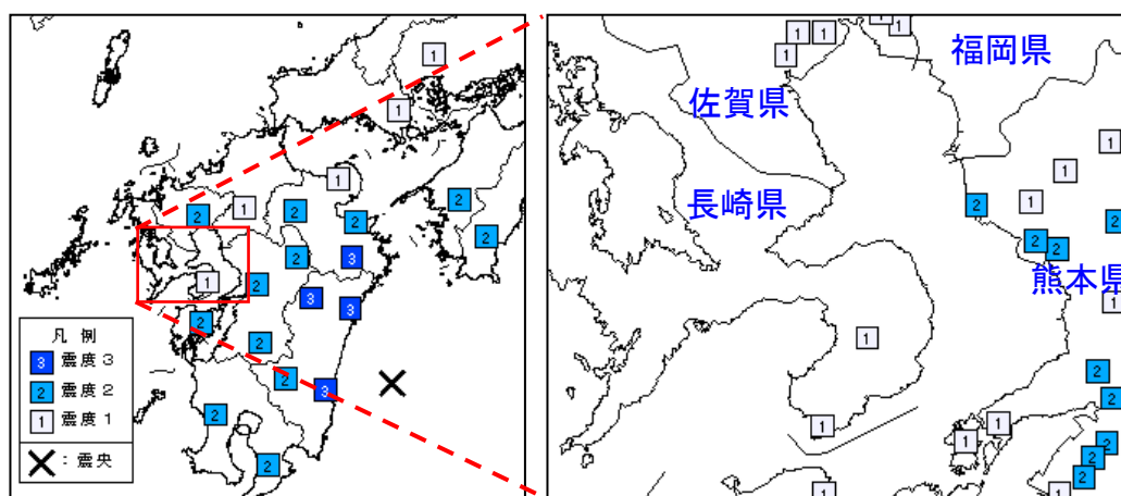
8月2日04時10分 M5.3 図4 震度分布図（左：地域別 右：観測点別）
