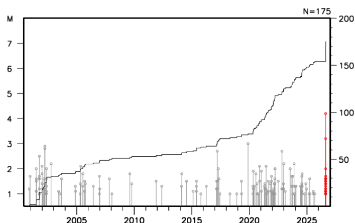
図10 図9領域d内の地震活動経過図及び回数積算図
