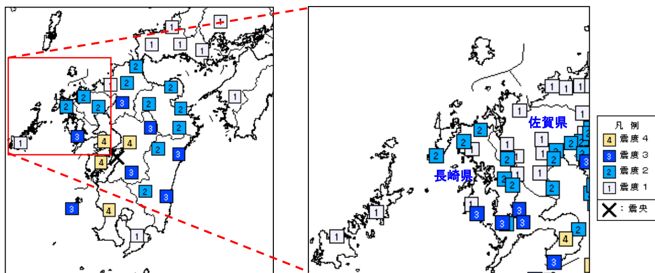
8 月 6 日 07 時 59 分 M5.1 図 1 震度分布図（左：地域別 右：市区町村別）
