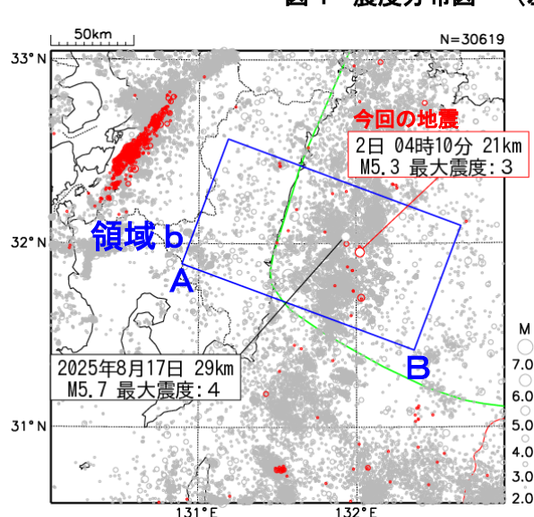
図5 震央分布図
