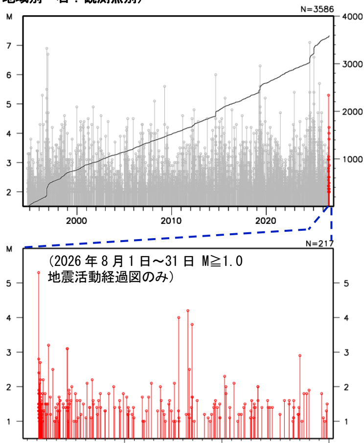
図7 図6領域c内の地震活動経過図及び回数積算図
