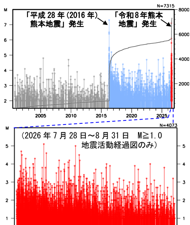
図 3 図 2 領域 a 内の地震活動経過図及び回数積算図
