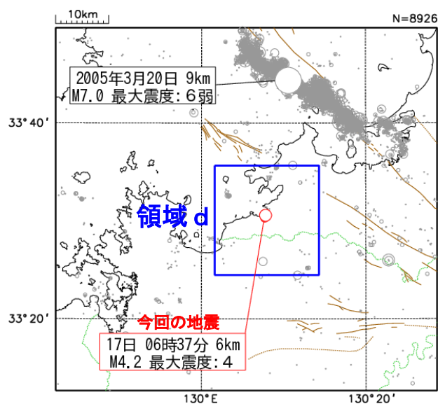
図9 震央分布図
