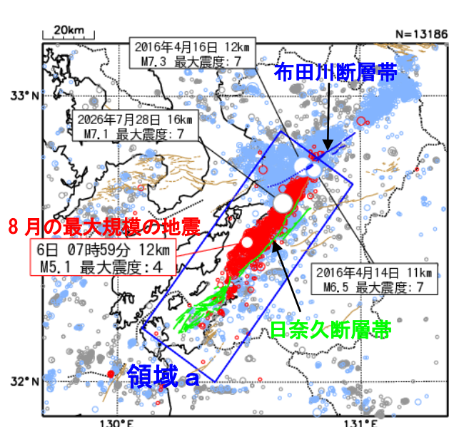
図 2 震央分布図
