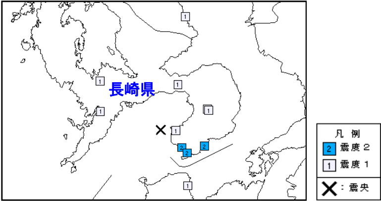
7 月 28 日 16 時 51 分 M3.0
