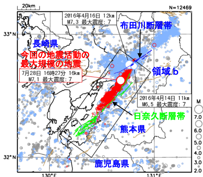
図 5 震央分布図
