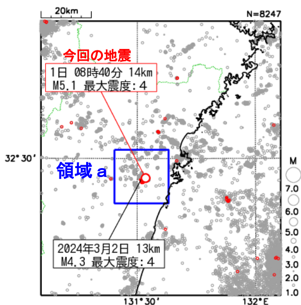
図 2 震央分布図
