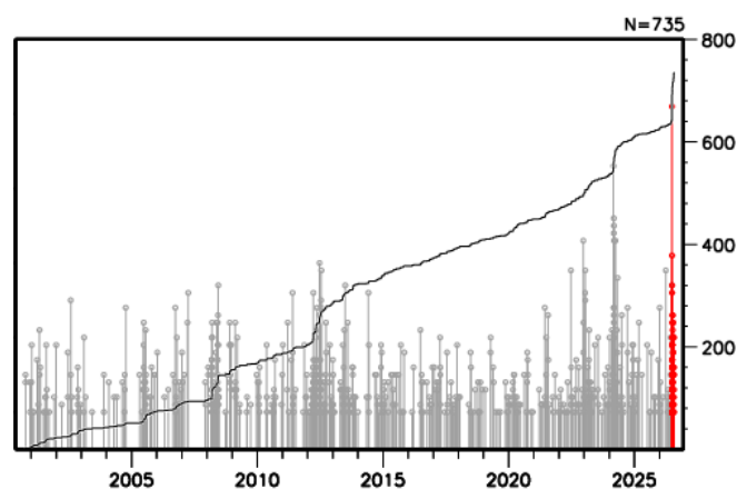
図 3 図 2 領域 a 内の地震活動経過図及び回数積算図
