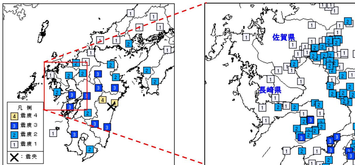
図 1 震度分布図（左：地域別、右：観測点別）
