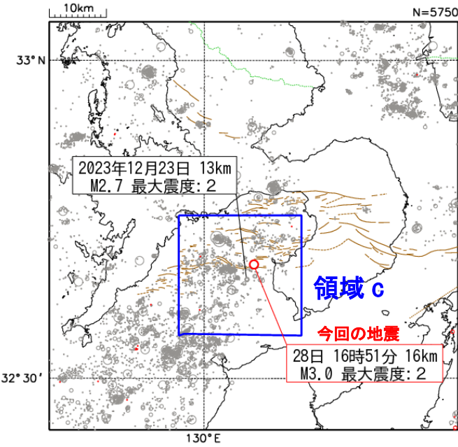
図 8 震央分布図
