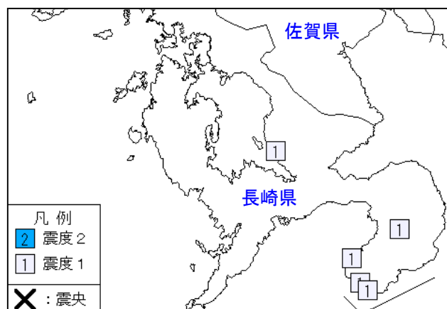
9月2日08時42分 M3.6 図1 震度分布図（観測点別）
