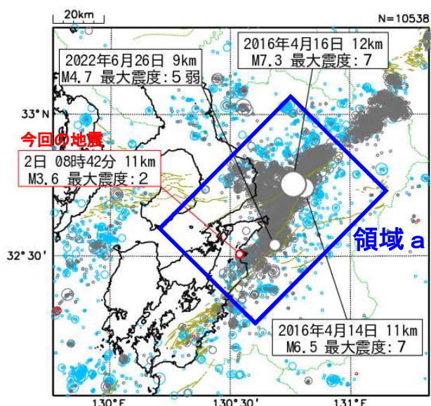
図2 震央分布図
