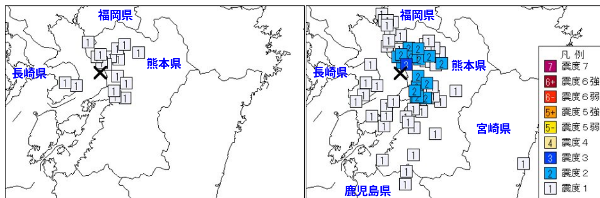
3月13日 00時23分 M3.2 3月13日 07時15分 M3.8 図1 震度分布図（観測点別、×：震央）
