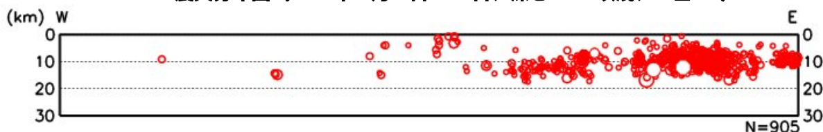
断面図（2020年3月1日～31日、深さ30km以浅、 M \geq 0.0 ） （震央分布図を南の方から見た断面図です）
