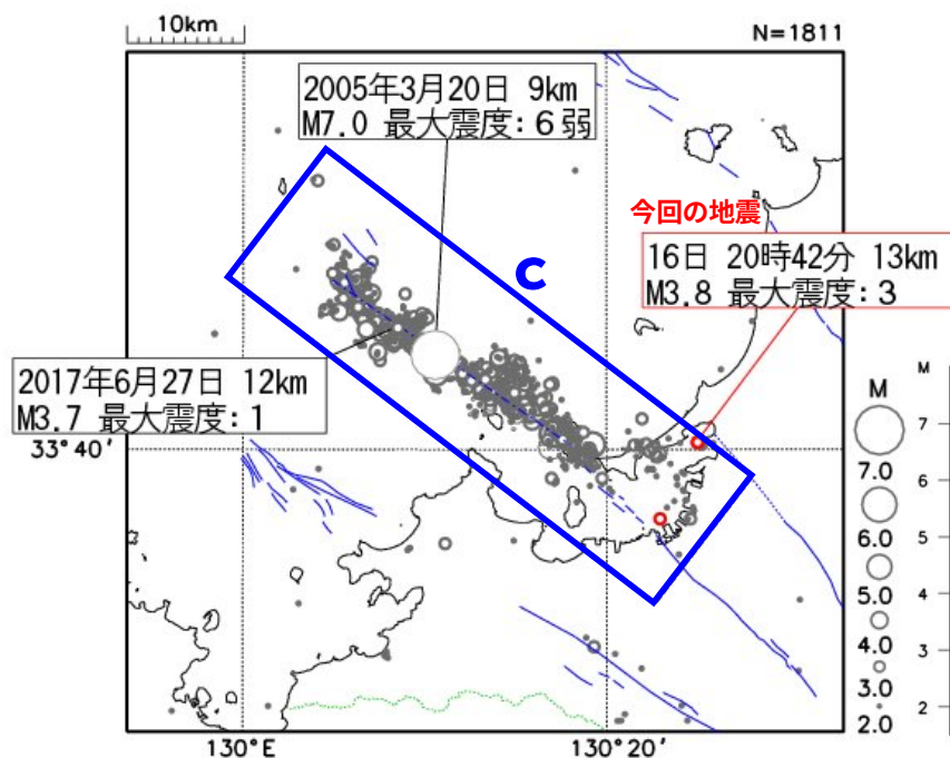
図8 震央分布図 (1997年10月1日～2020年3月31日 深さ0km～30km M \geq 2.0)
