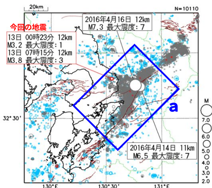
図2 震央分布図
