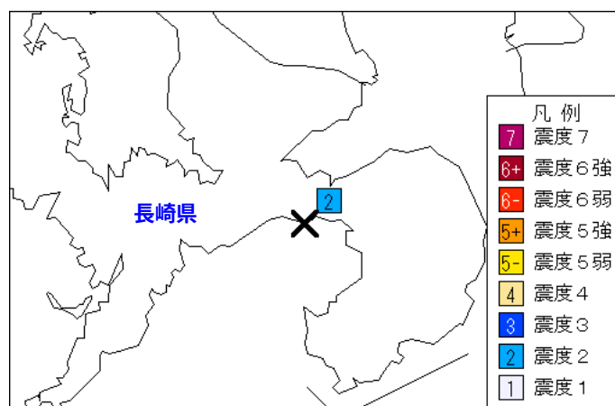
3月13日 12時59分 M2.4 図4 震度分布図（観測点別、×：震央）
