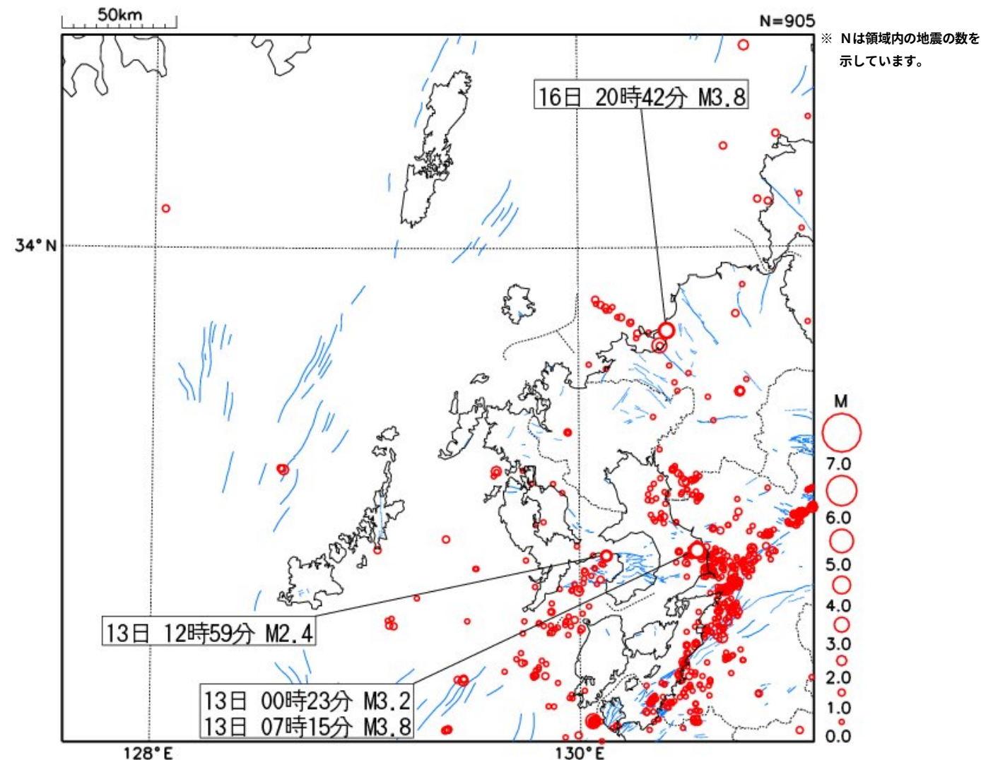
震央分布図（2020年3月1日～31日、深さ30km以浅、 M \geq 0.0 ）
