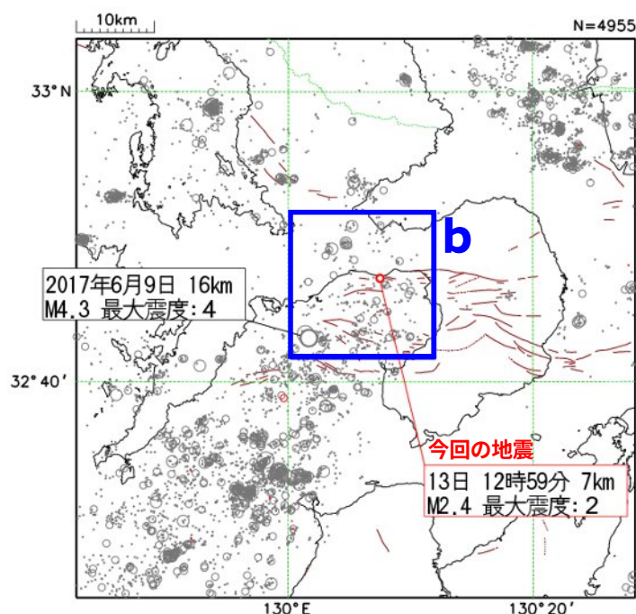
図5 震央分布図 (1997年10月1日～2020年3月31日 深さ0km～20km M \geq 1.0)
