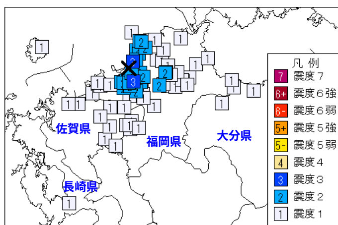
3月16日 20時42分 M3.8 図7 震度分布図（観測点別、×：震央）
