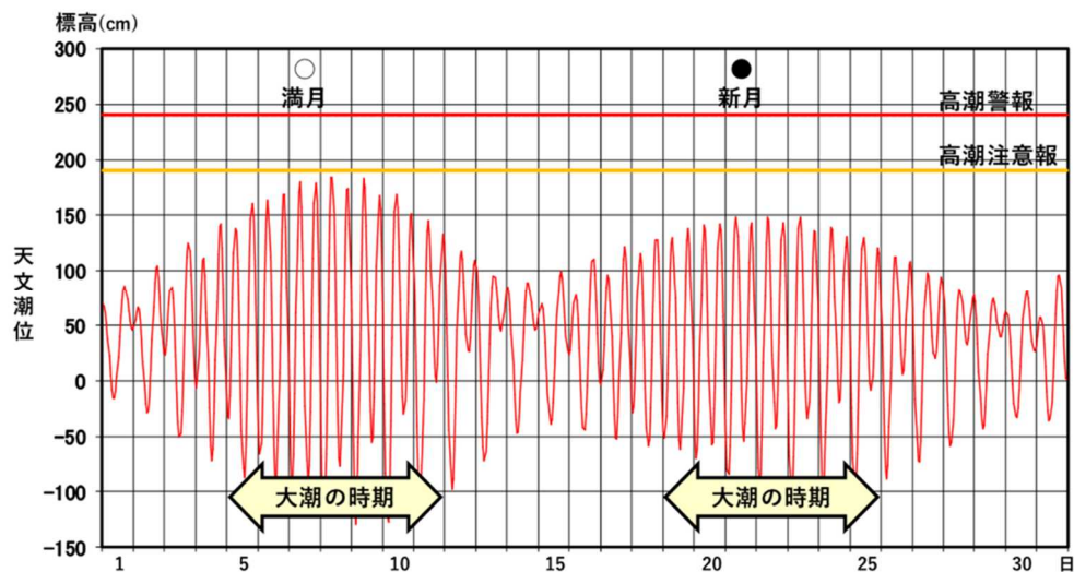
図3 長崎における2025年10月（1時間ごとの）の天文潮位
