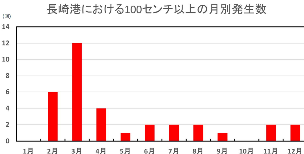
図2 長崎港における1997年~2023年での100 cm以上の「あびき」の月別発生回数
