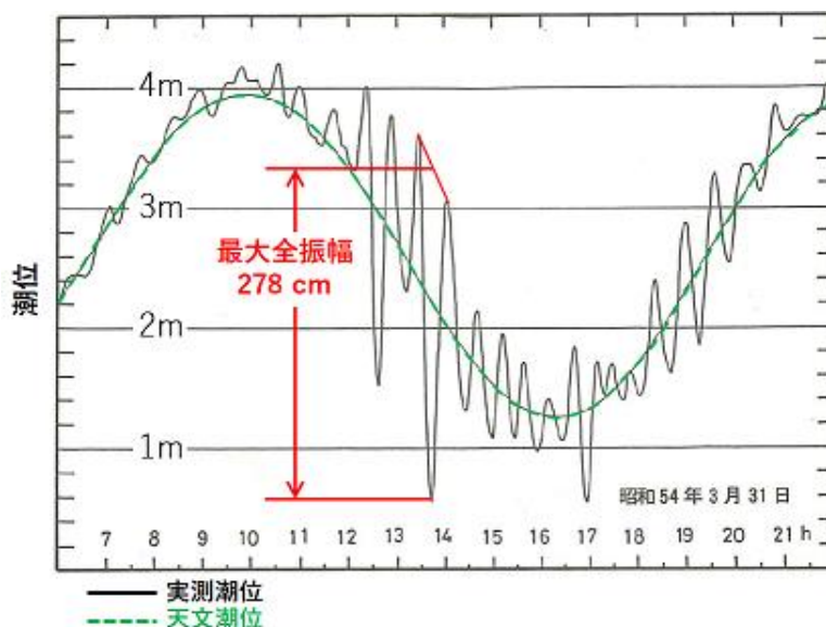
図1 1979年(昭和54年)3月31日の長崎検潮所における天文潮位(緑)と副振動(あびき)(黒)の例
