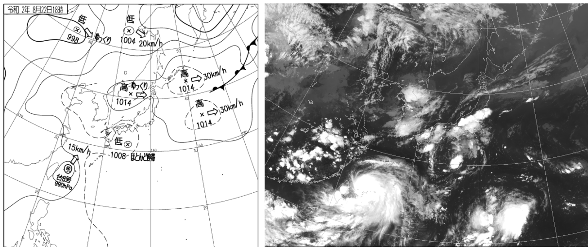
8月22日18時の地上天気図(左)と気象衛星赤外面像(右)
