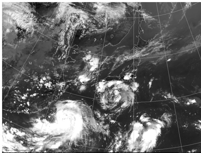
8月22日15時の地上天気図(左)と気象衛星赤外面像(右)
