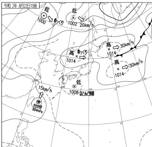
8月22日15時の地上天気図(左)と気象衛星赤外面像(右)
