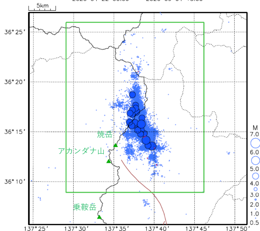
震央分布図 深さ0~20 km M \geq 0.5
