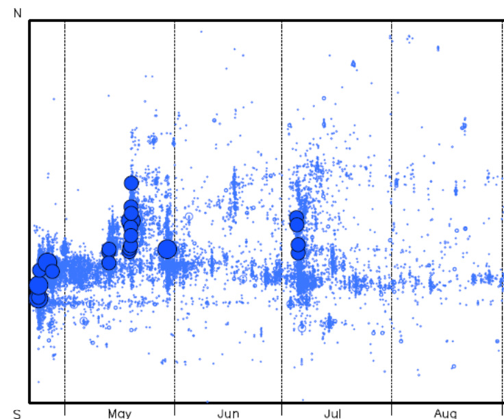
震央分布図の矩形内のMT図及び回数積算図
