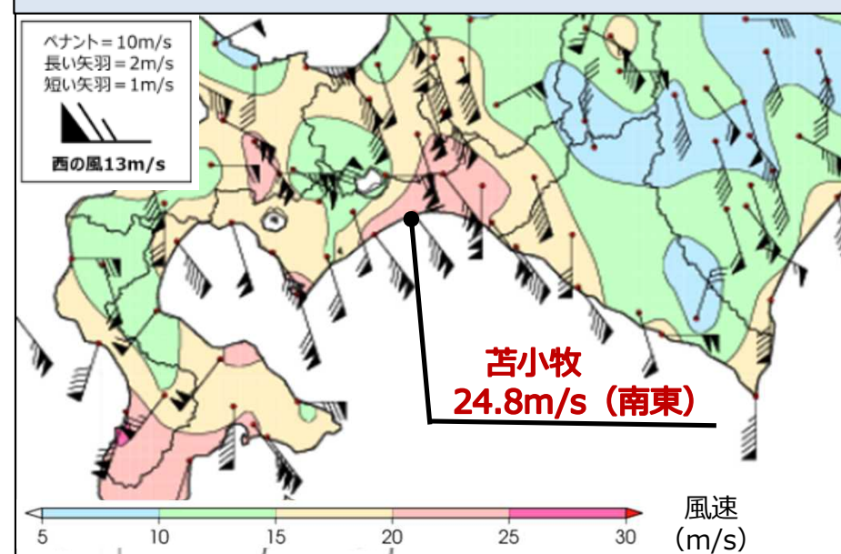
13日の日最大瞬間風速
