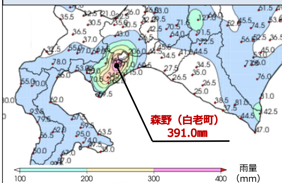
14日06時までの24時間雨量
