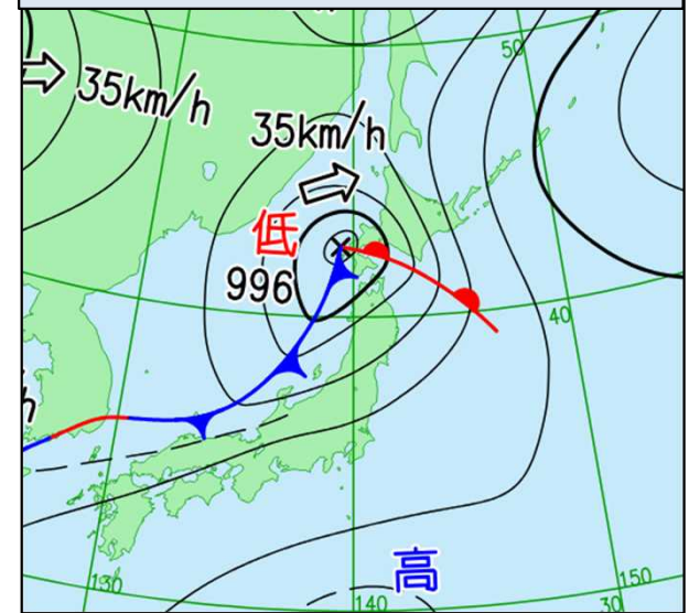
地上天気図（13日21時）
