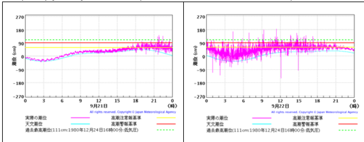
宮古（臨時）[気象庁]の潮位の実況（平成23年9月21日00時～9月22日24時）
