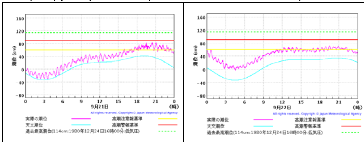
大船渡（臨時）[気象庁]の潮位の実況（平成23年9月21日00時～9月22日24時）
