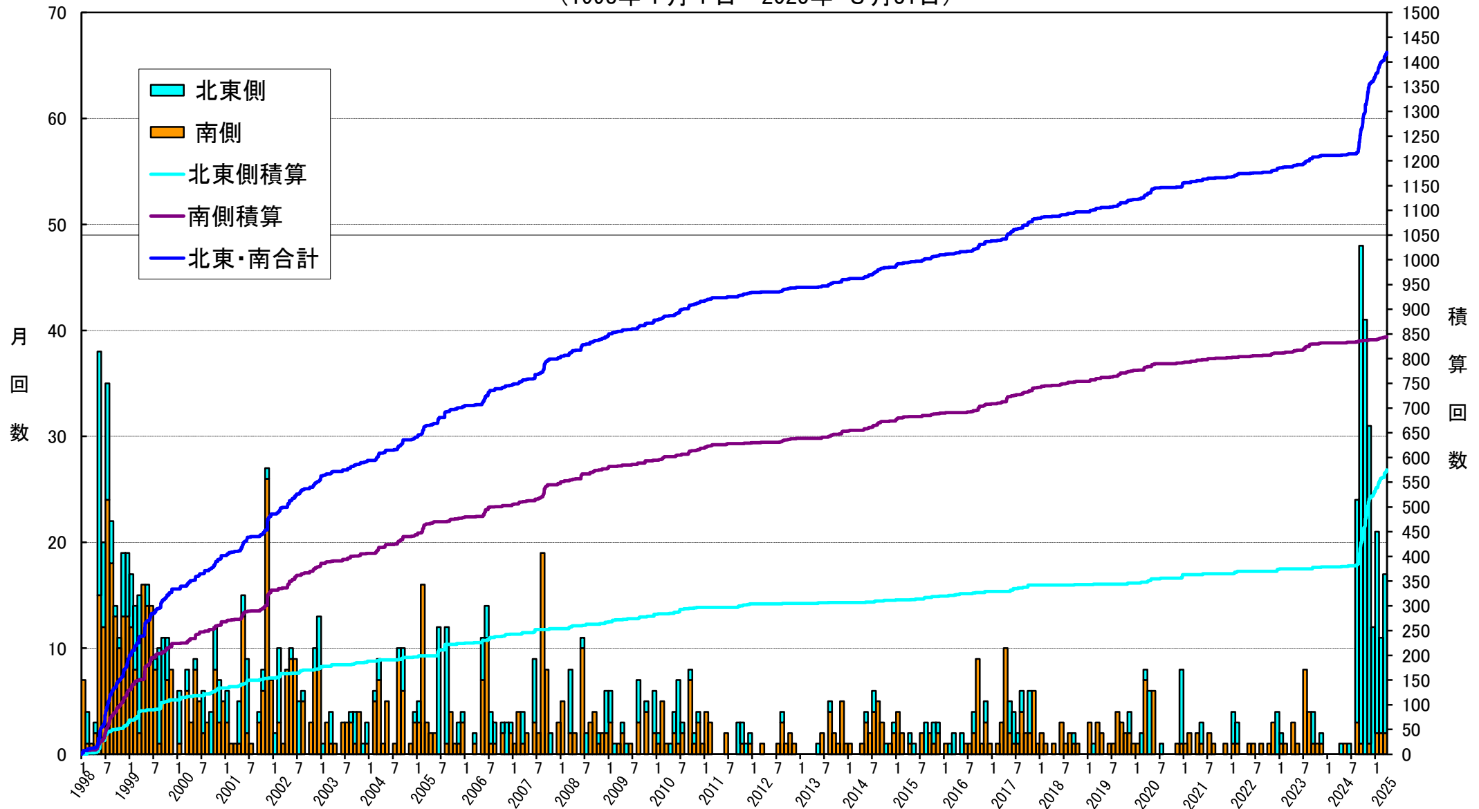
岩手山周辺で発生した深部低周波地震の月別回数と積算回数 (1998年1月1日～2025年3月31日)
