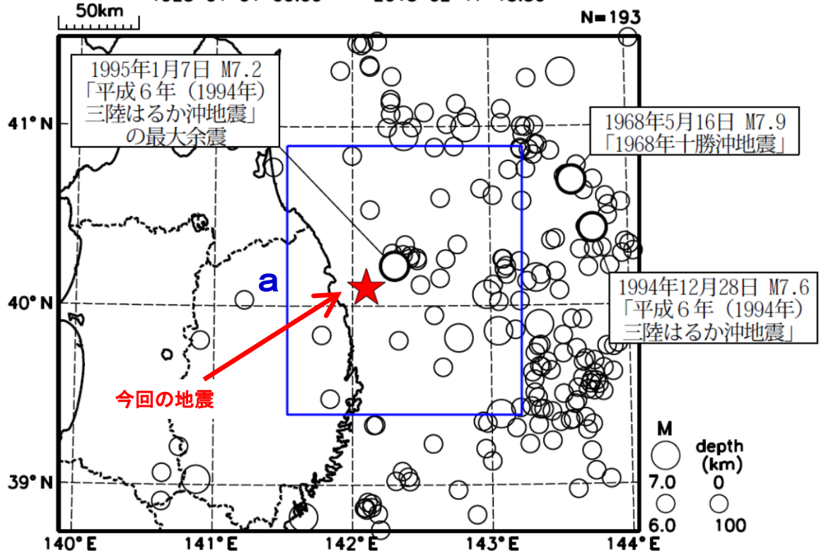
震央分布図
