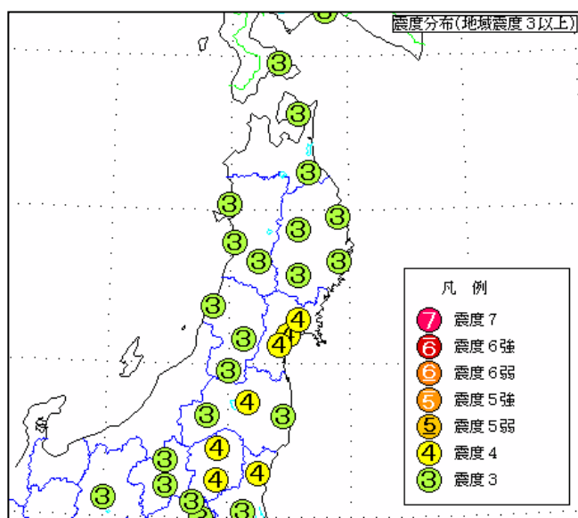
地域毎の震度分布図
