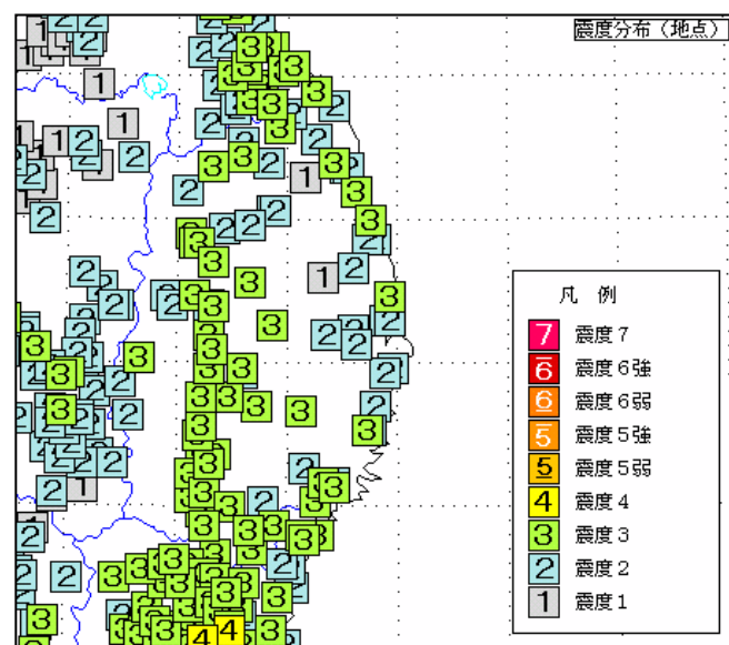
観測点毎の震度分布図（県内拡大図）
