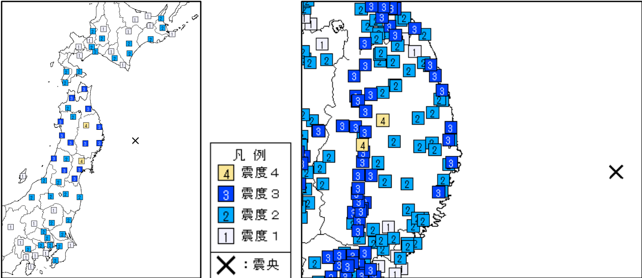
図5. 震度分布図
