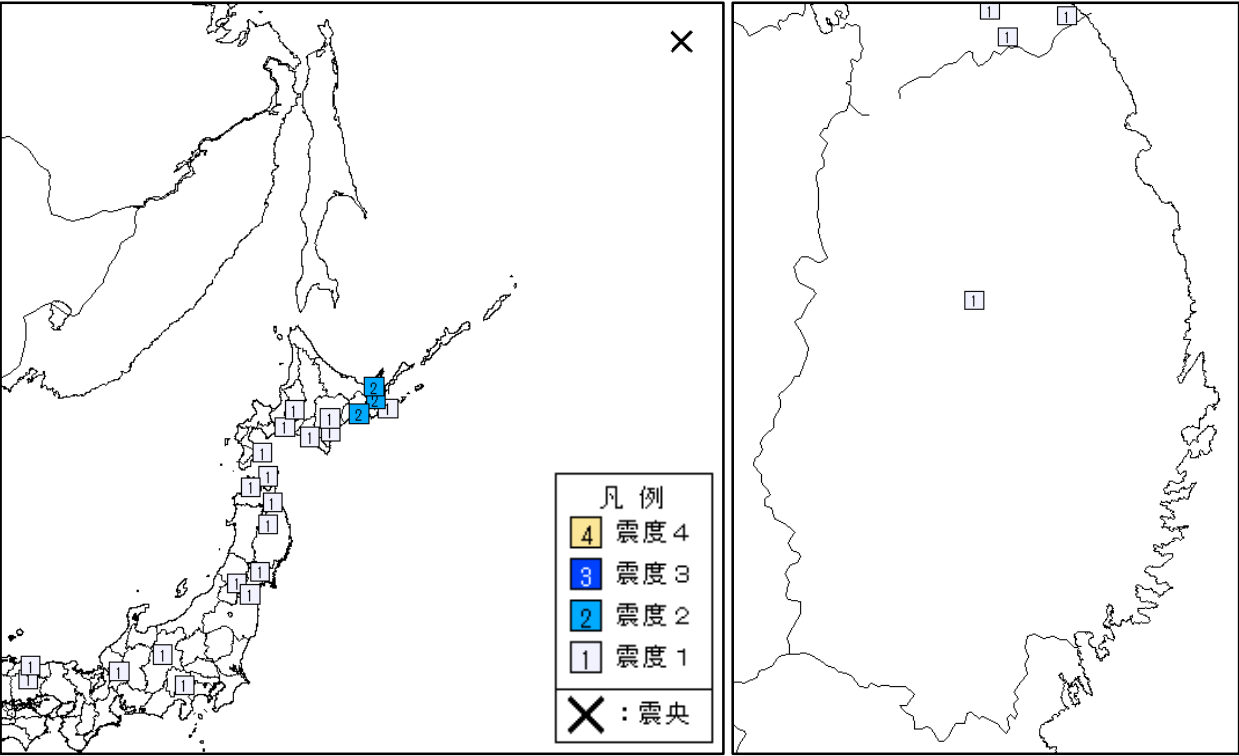
図3. 震度分布図
