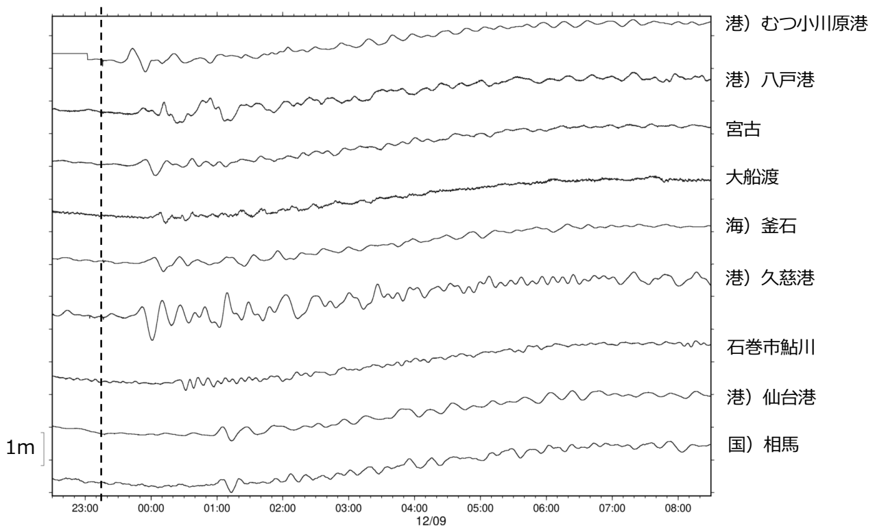
図7．2025 年 12 月 8 日 23 時 15 分に発生した青森県東方沖の地震による津波の観測波形（東北地方）
