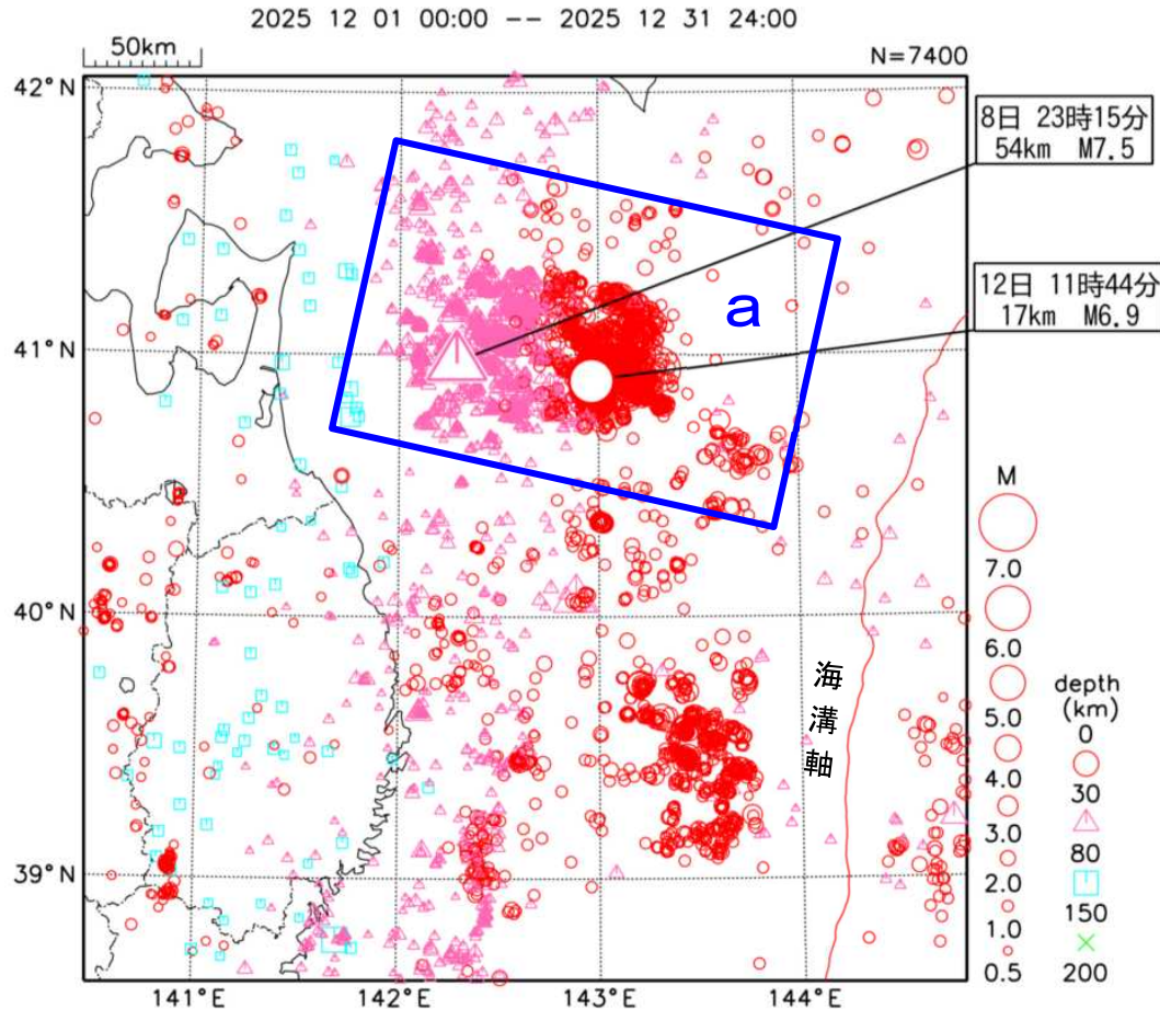
図3. 震央分布図
