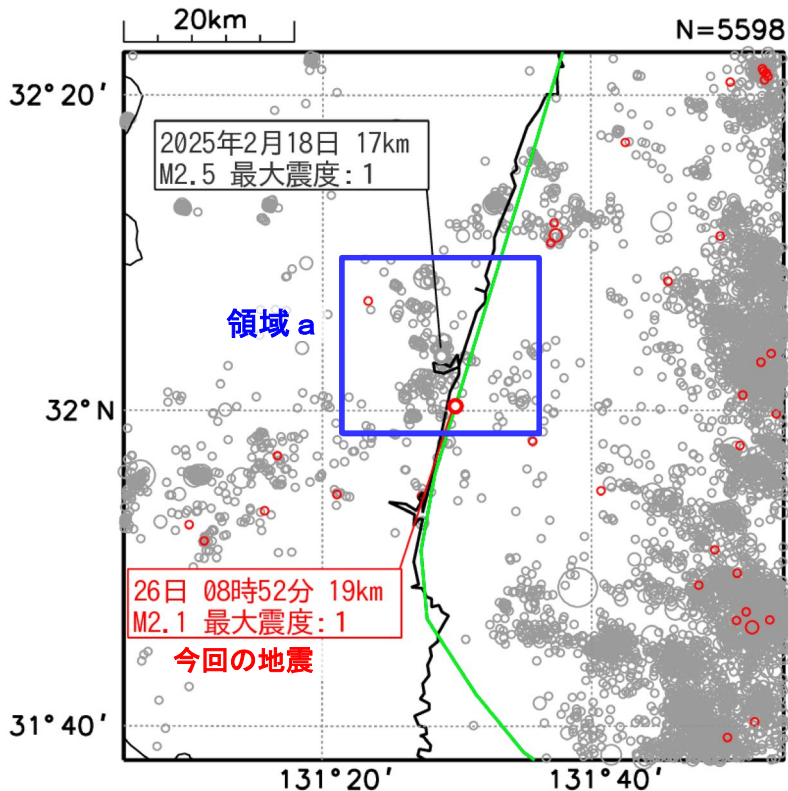
図 12 震央分布図
