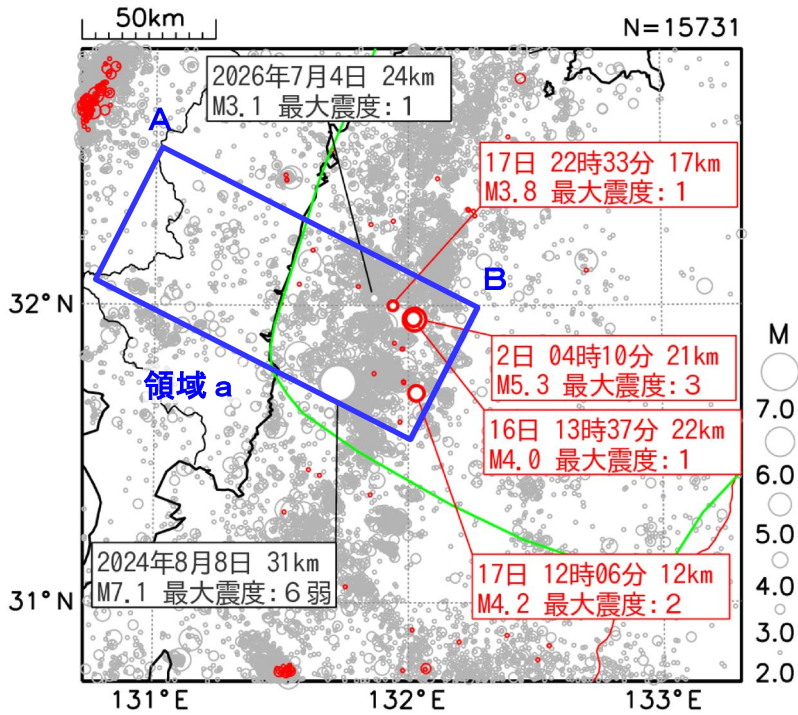
図5 震央分布図 (1997年10月1日～2026年8月31日、 深さ0～100km、 M \geq 2.0 ) ※2026年8月の地震を赤色で表示 緑色の線は南海トラフ巨大地震の想定震源域を示しています。
