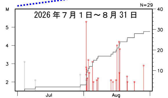
図7 図6領域b内の地震活動経過図 および回数積算図
