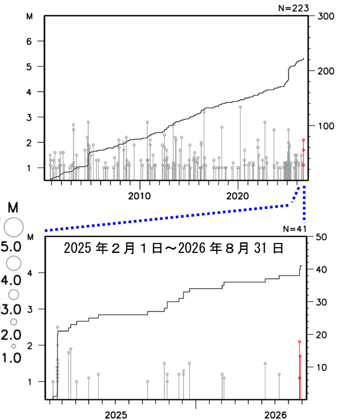
図 13 図 12 領域 a 内の地震活動経過図 および回数積算図
