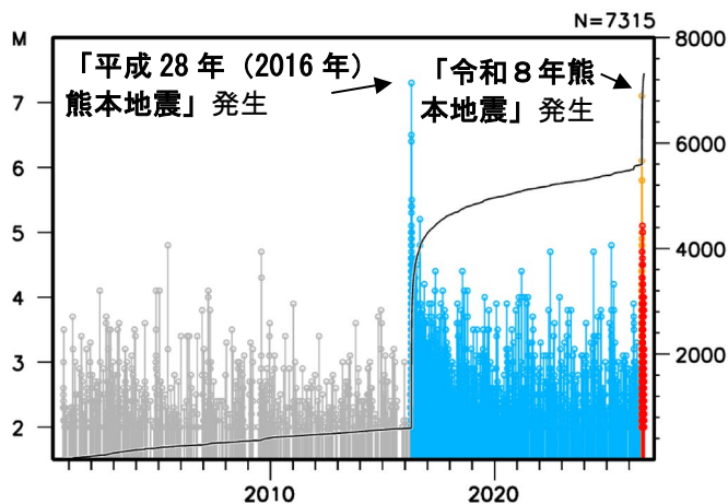
図 3 図 2 領域 a 内の地震活動経過図および回数積算図
