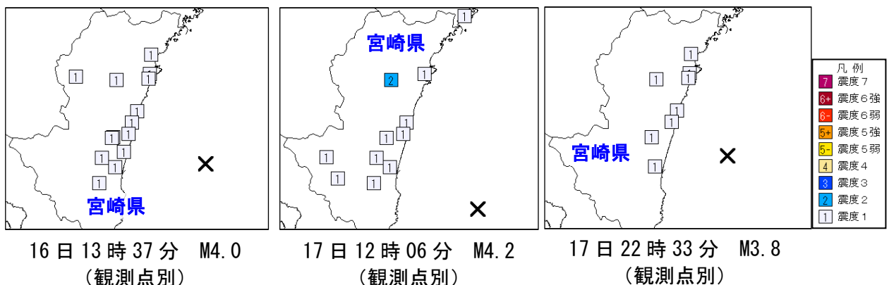
図4 震度分布図（×：震央）
