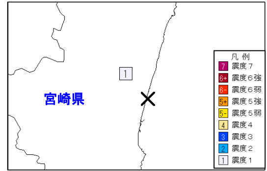
図 11 震度分布図（観測点別、×：震央）
