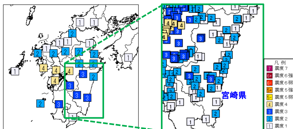
12 日 13 時 05 分 M5.0 熊本県天草・芦北地方 （左図：地域別、右図：観測点別）
