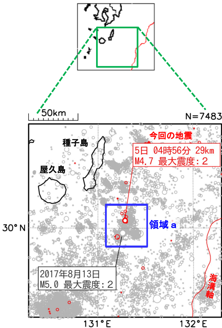
図9 震央分布図 (1997年10月1日～2026年8月31日、 深さ0～80km、 M \geq 2.5 ) ※2026年8月の地震を赤色で表示
