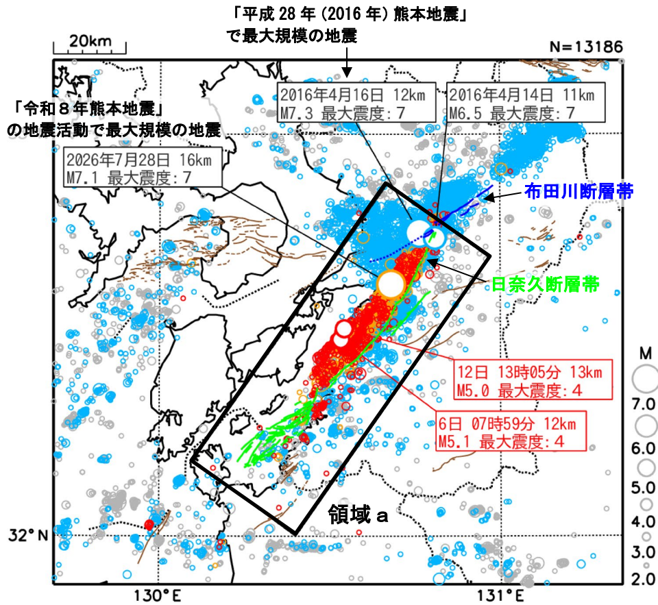
図 2 震央分布図
