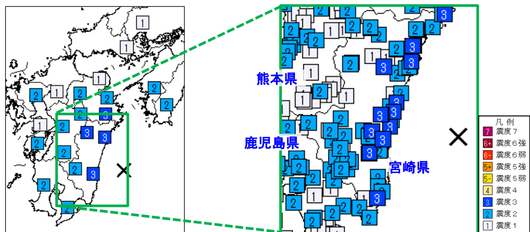
2日04時10分 M5.3（左図：地域別、右図：観測点別）
