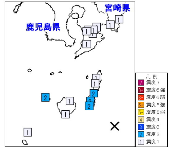
図8 震度分布図（観測点別、×：震央）
