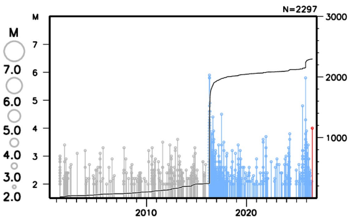
図 20 図 19 領域 a 内の地震活動経過図 および回数積算図
