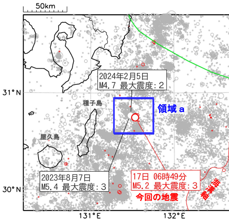
図 13 震央分布図
