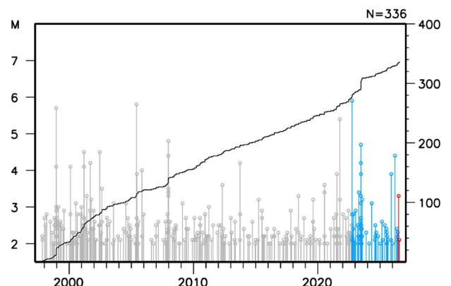
図7 図6領域b内の地震活動経過図 および回数積算図
