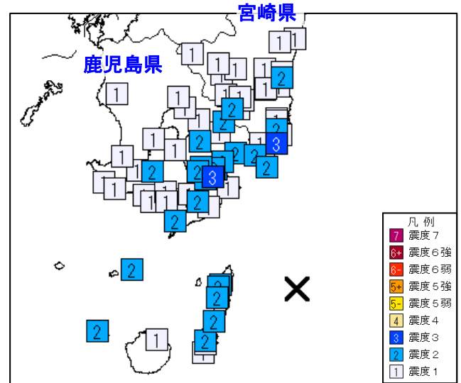
図 12 震度分布図（観測点別、×：震央）
