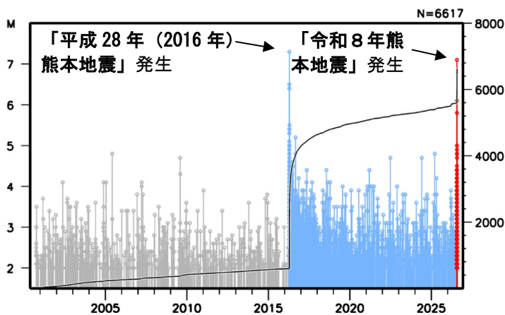
図 17 図 16 領域 a 内の地震活動経過図 および回数積算図
