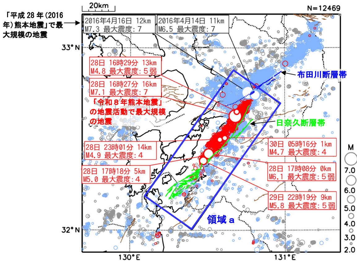
図 16 震央分布図
