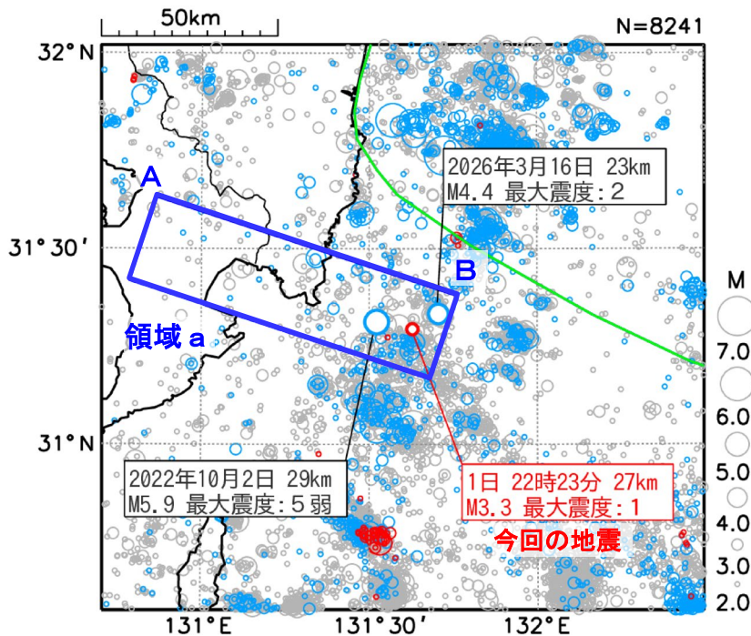
図5 震央分布図
