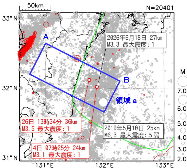
図9 震央分布図
