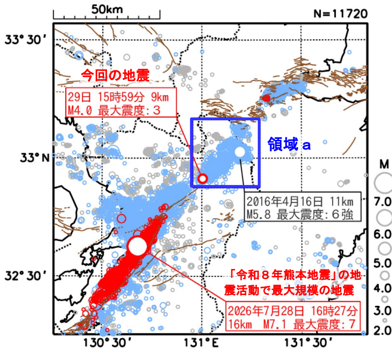
図 19 震央分布図
