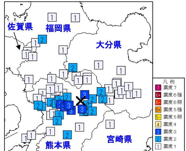
図 18 震度分布図（観測点別、×：震央）
