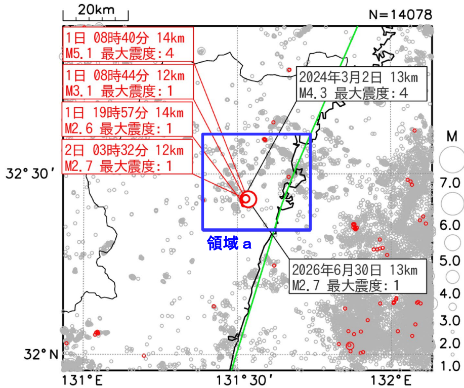
図2 震央分布図
