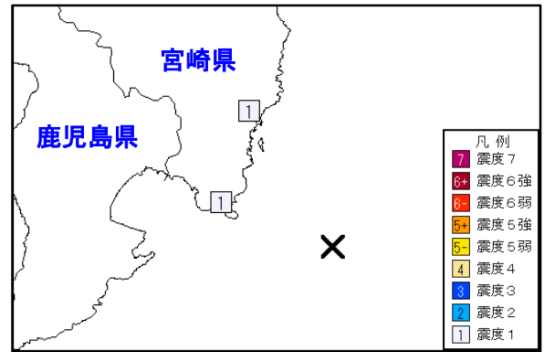
図4 震度分布図(観測点別、×:震央)
