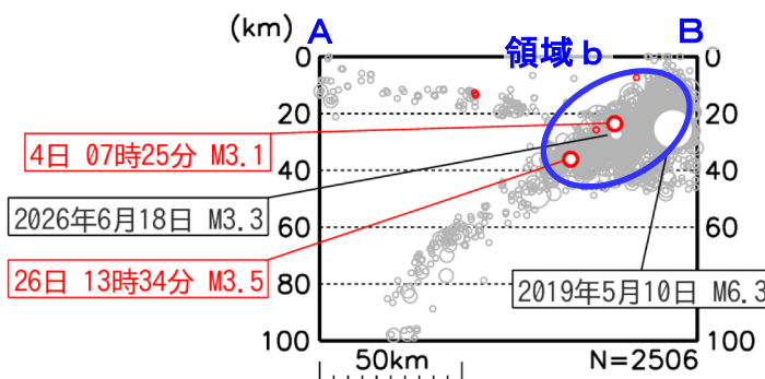
図10 図9領域a内の断面図(A-B投影)
