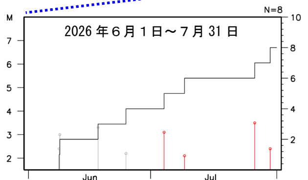
図11 図10領域b内の地震活動経過図 および回数積算図
