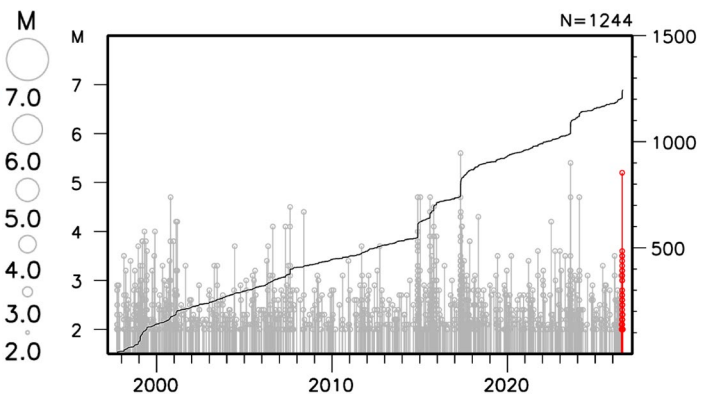
図 14 図 13 領域 a 内の地震活動経過図 および回数積算図
