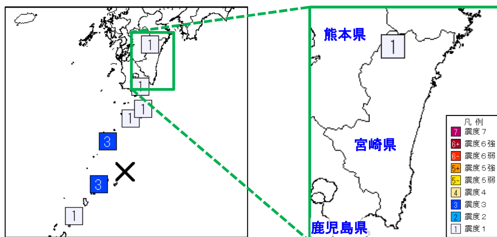
図1 震度分布図（左図：地域別、右図：観測点別、×：震央）
