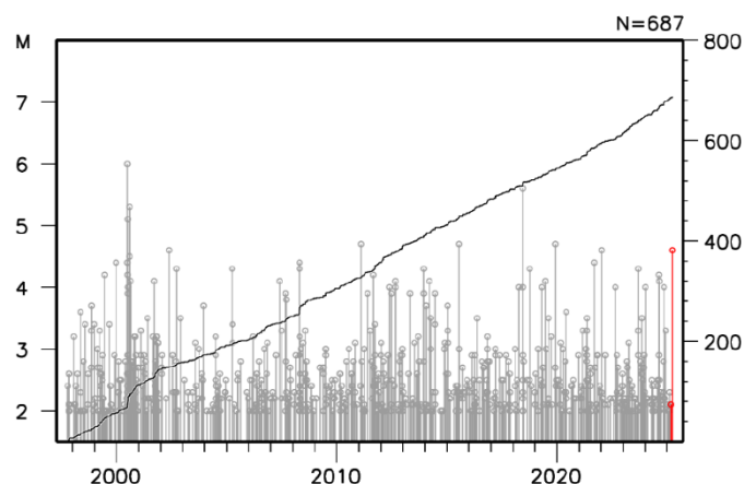
図 10 図 9 領域 b 内の地震活動経過図 および回数積算図
