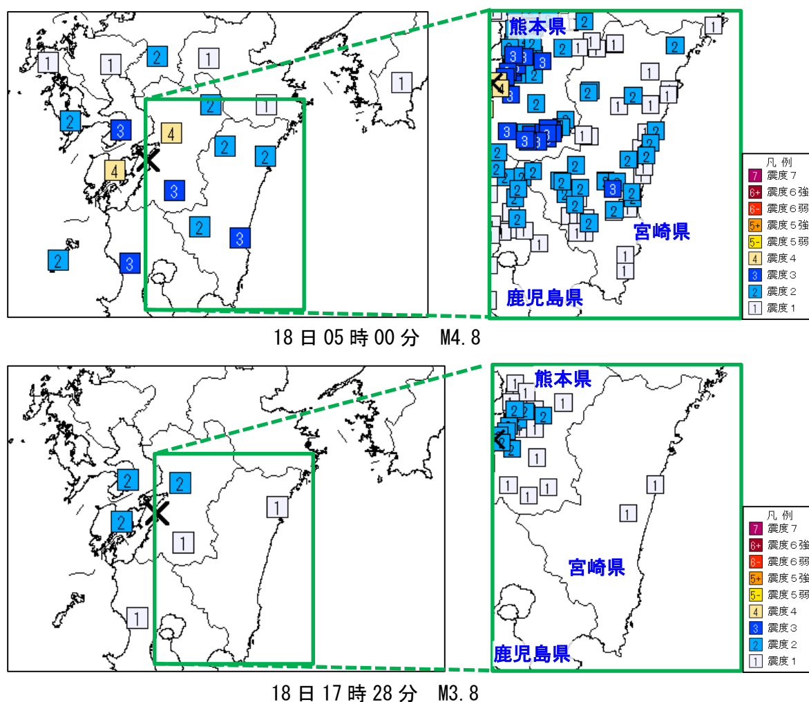
図 4 震度分布図（左図：地域別、右図：観測点別、×：震央）
