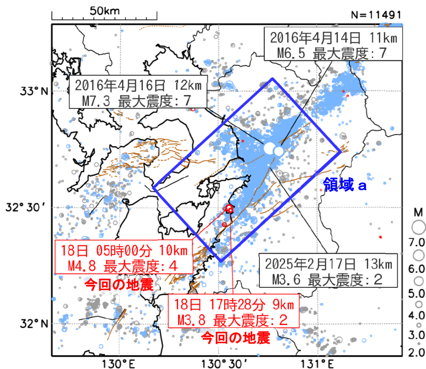
図5 震央分布図
