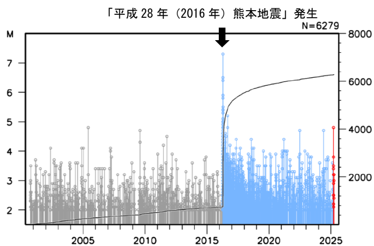
図6 図5領域a内の地震活動経過図 および回数積算図
