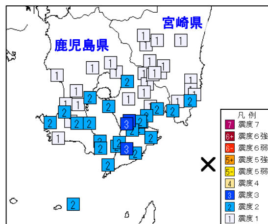
図 7 震度分布図（観測点別、×：震央）
