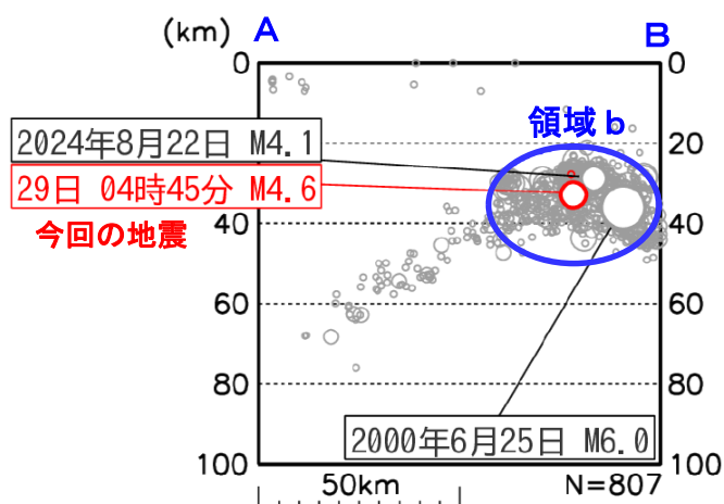
図 9 図 8 領域 a 内の断面図（A－B 投影）
