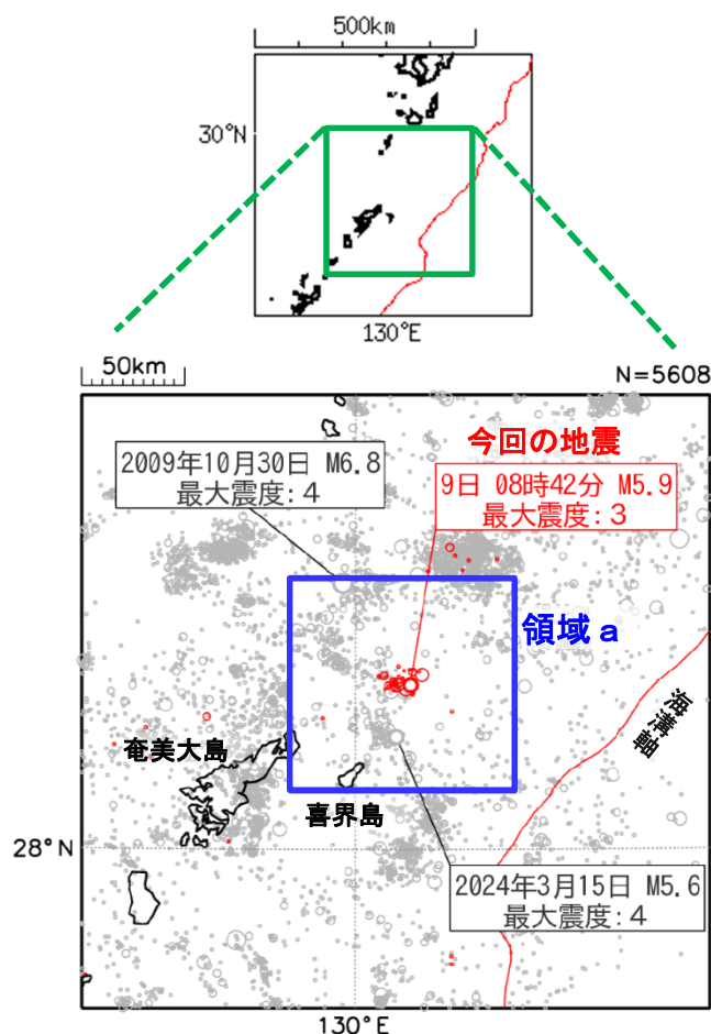
図2 震央分布図
