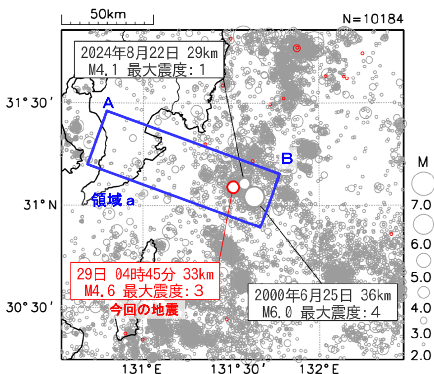
図 8 震央分布図
