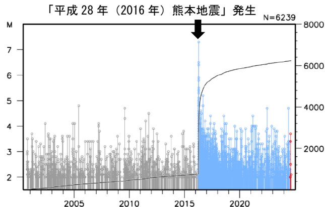
図 8 図 7 領域 a 内の地震活動経過図および回数積算図
