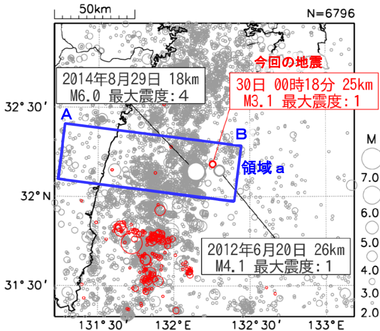
図 17 震央分布図
