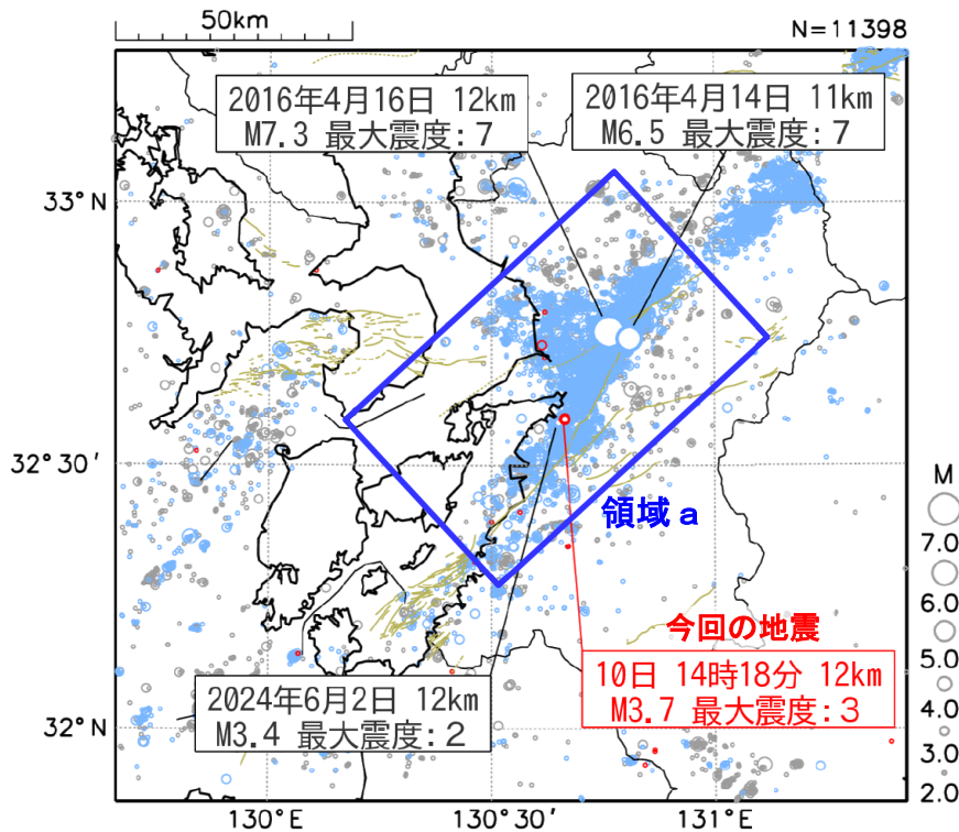
図 7 震央分布図
