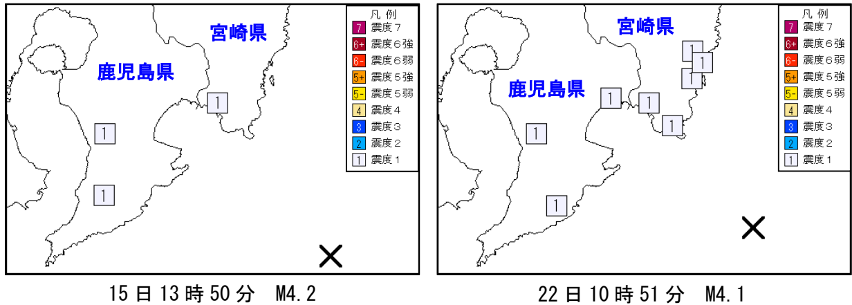
図 12 震度分布図（観測点別、×：震央）
