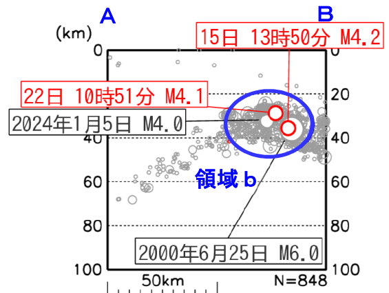
図 14 図 13 領域 a 内の断面図（A－B 投影）
