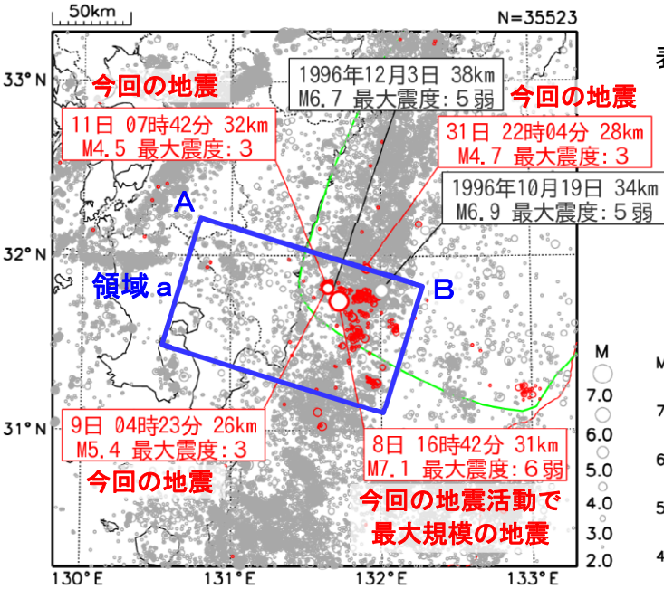
図3 震央分布図 (1994年10月1日～2024年8月31日、 深さ0～100km、M≥2.0)
