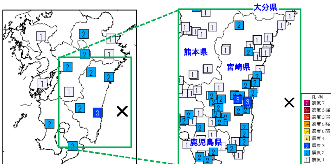
図 1 震度分布図 (県内で震度 3 以上を観測した地震、左：地域別、右：観測点別、×：震央)
