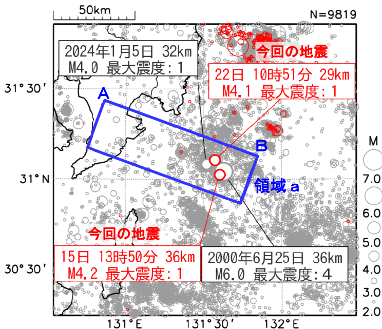
図 13 震央分布図
