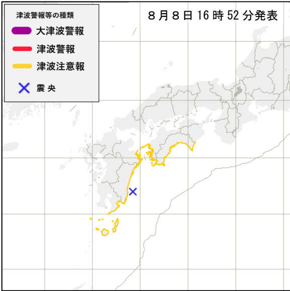
図2 8月8日の日向灘の地震に対して発表した津波注意報
