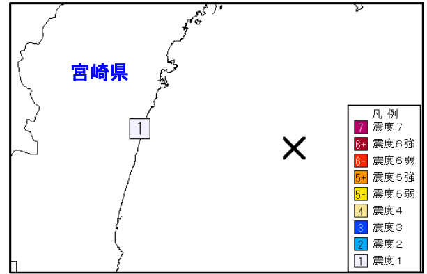
図 16 震度分布図（観測点別、×：震央）
