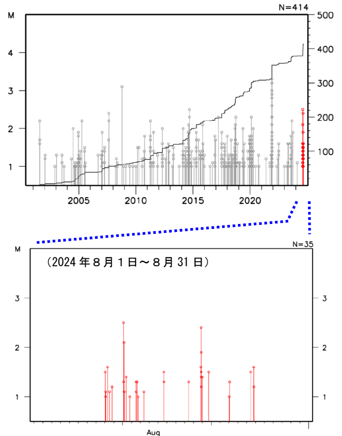
図 11 図 10 領域 a 内の地震活動経過図
