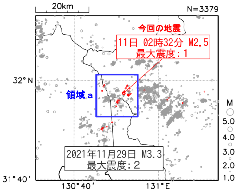
図 10 震央分布図 (2000 年 10 月 1 日～2024 年 8 月 31 日、 深さ 0～30km、 M \geq 1.0 ) 2024 年 8 月の地震を赤色で表示
