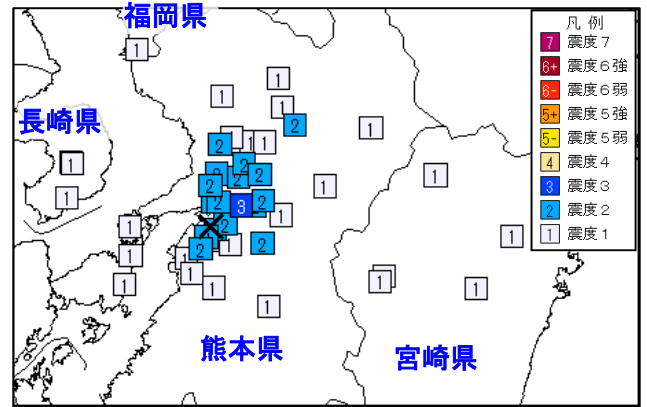
図 6 震度分布図（観測点別、×: 震央）
