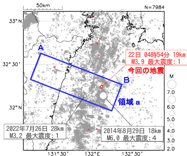
図 2 震央分布図
