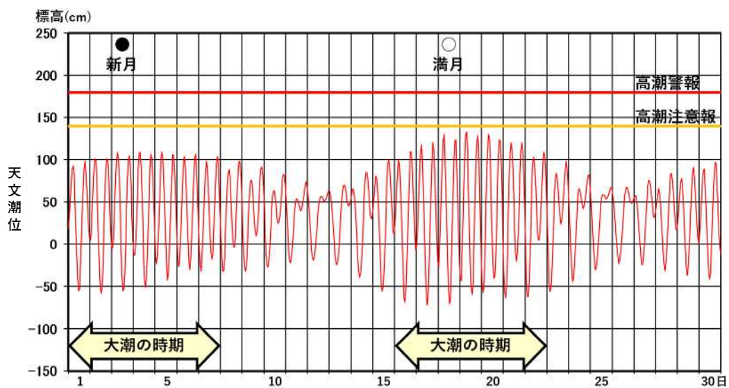
図3 油津における2024年9月(1時間ごとの)の天文潮位
