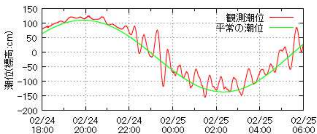
2009年2月24～25日に長崎で起こった副振動
