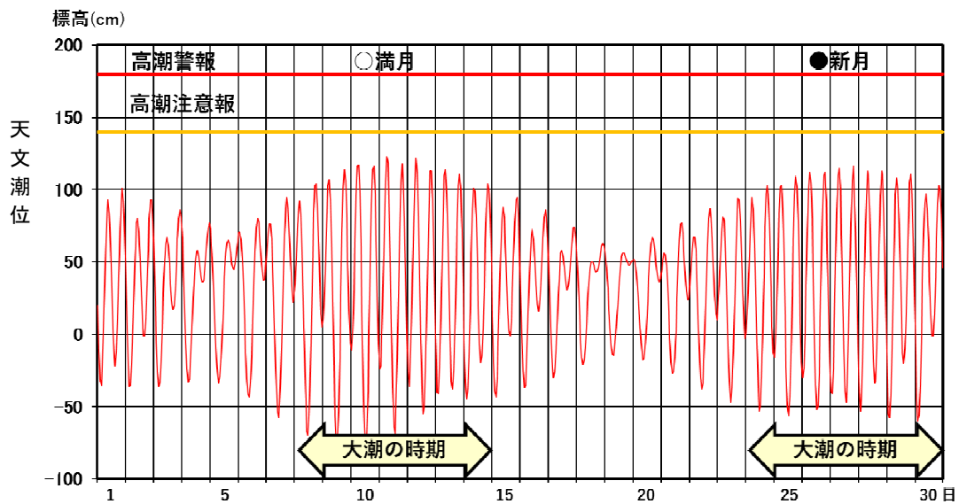
図3 油津における2022年9月（1時間ごとの）の天文潮位
