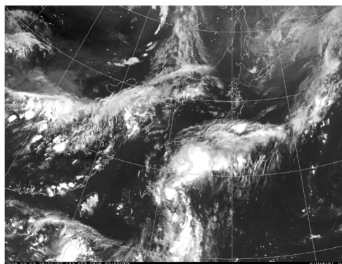
9月3日18時の地上天気図（左）と気象衛星赤外画像（右）
