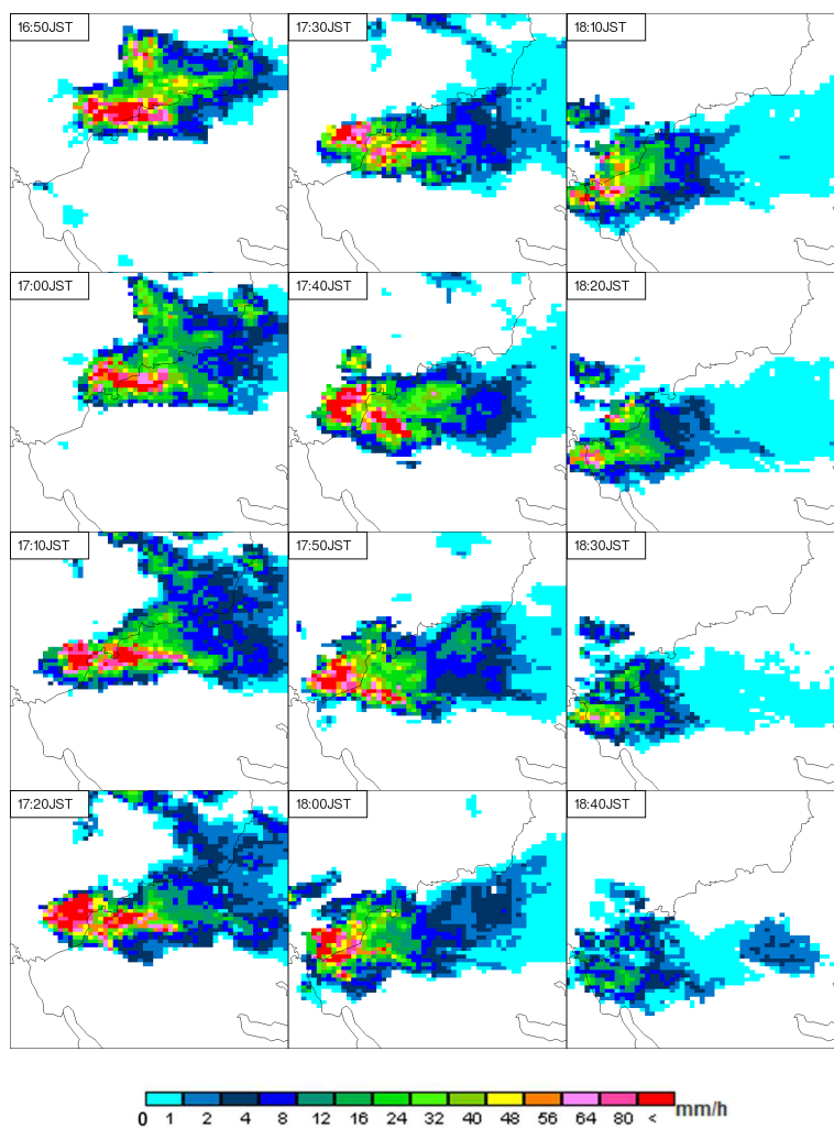
9月3日16時50分から10分毎のレーダー画像
