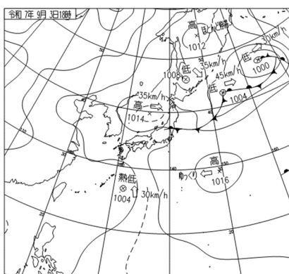
9月3日18時の地上天気図（左）と気象衛星赤外画像（右）
