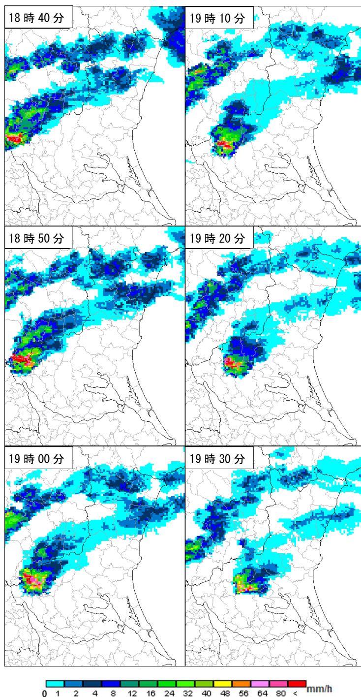
7月10日18時40分から10分毎のレーダー画像
