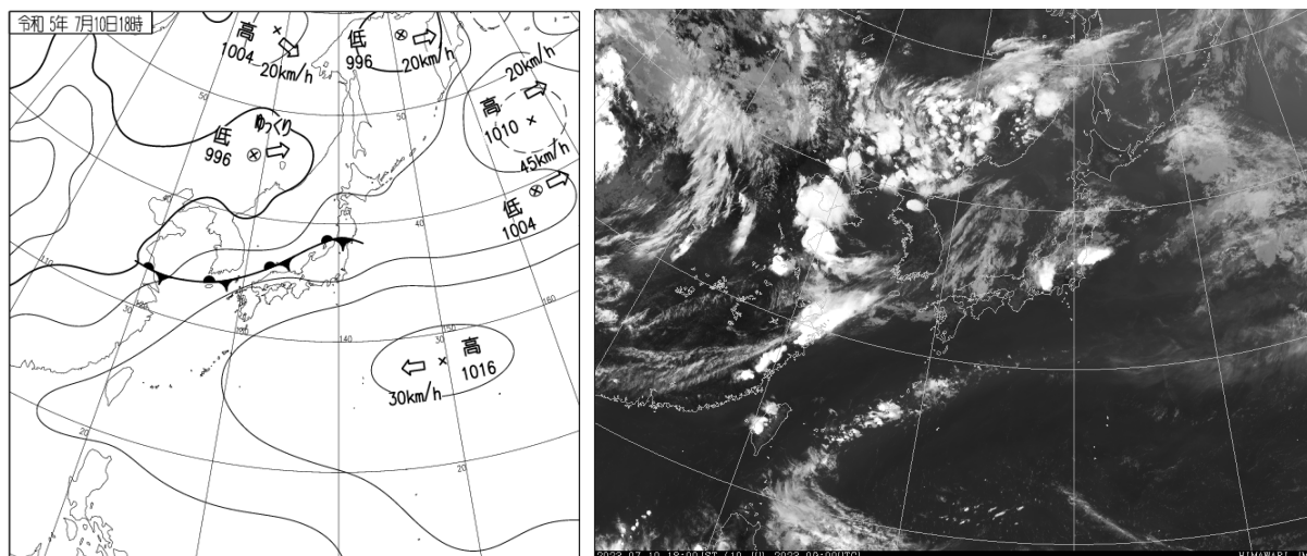
7月10日18時の地上天気図（左）と気象衛星赤外画像（右）
