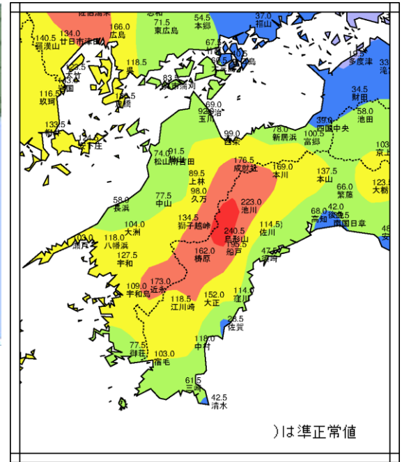
降水分布図(8月8日13時~9日14時)
