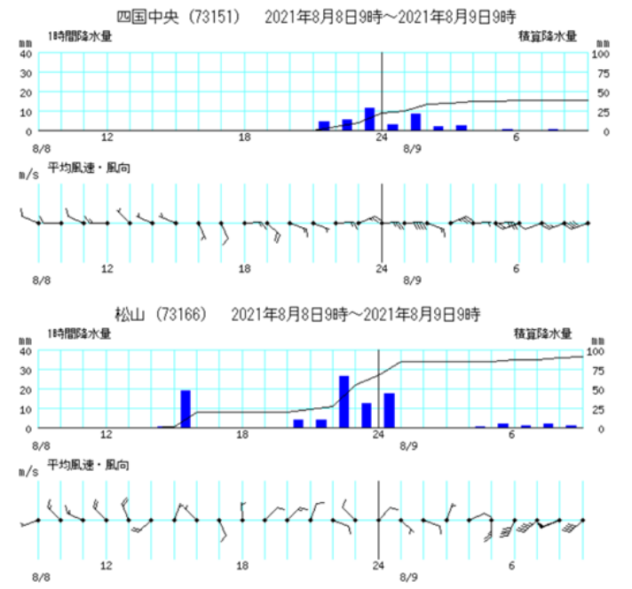
1時間降水量及び平均風速・風向時系列図 (8月8日09時~9日09時)
