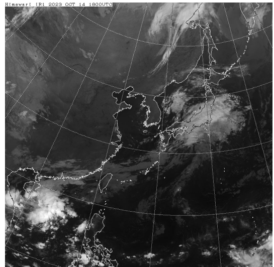
気象衛星赤外画像(10月15日03時)
