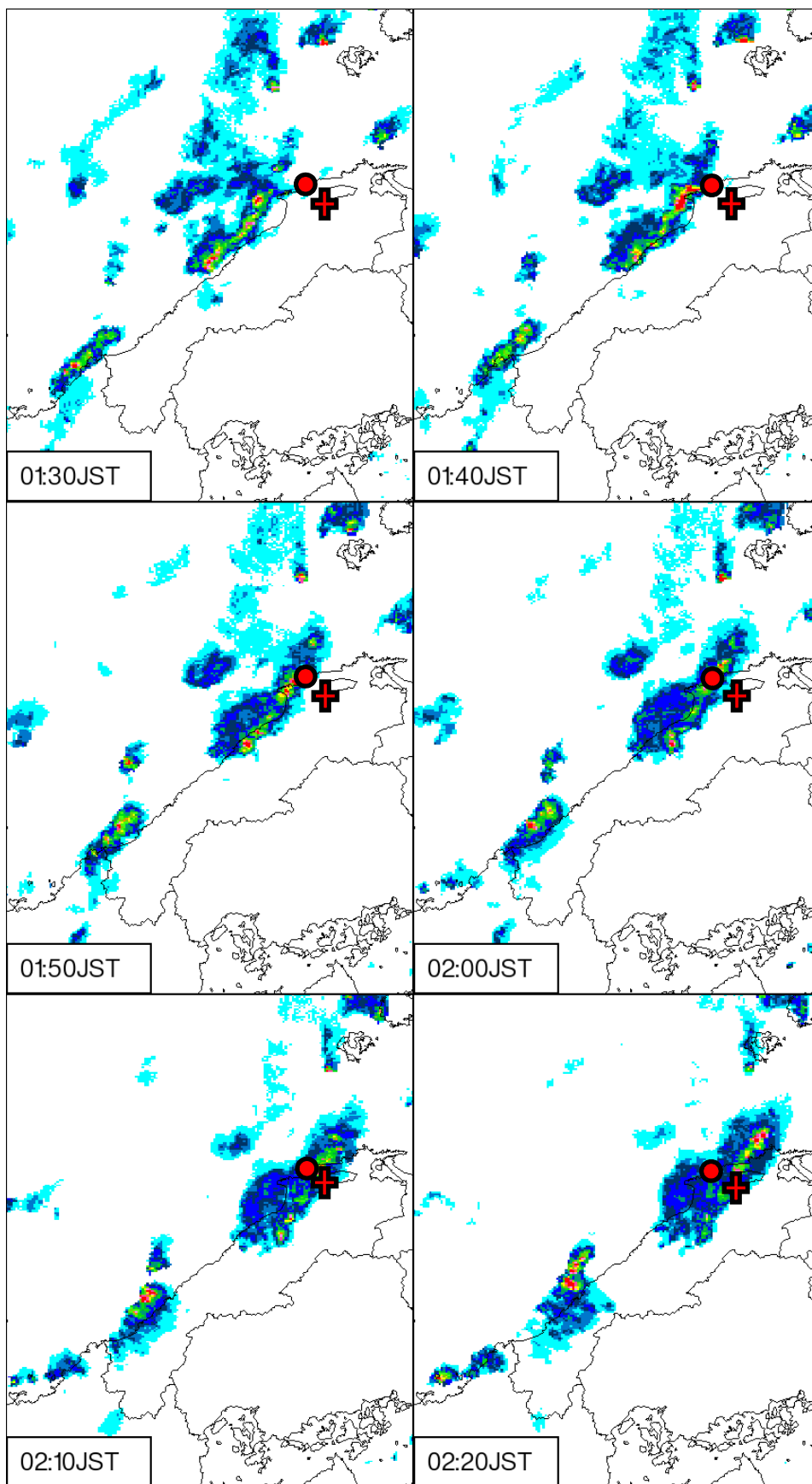
気象レーダー画像(降水強度) (10月15日01時30分～02時20分)
