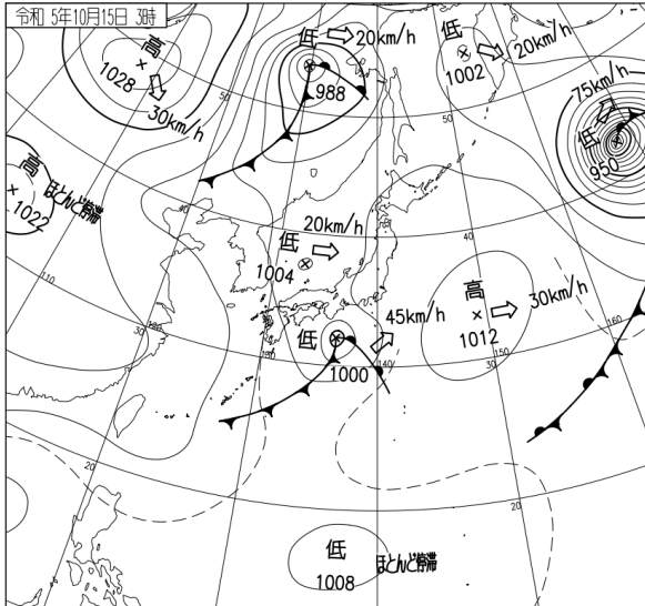
地上天気図(10月15日03時)
