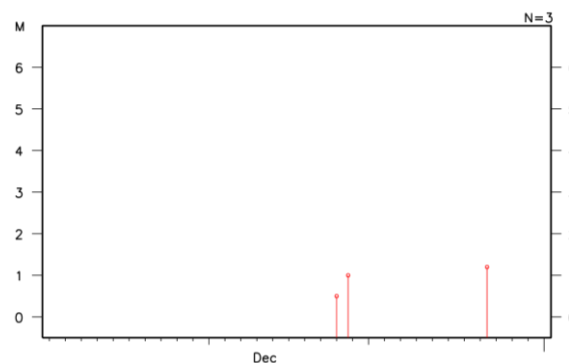
図 3 地震活動経過図（図 2 の領域内）
