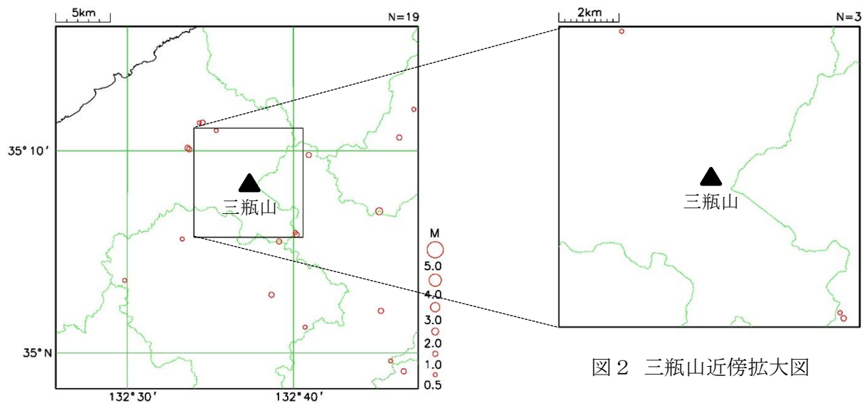
図1 三瓶山周辺の震央分布図 (2025年6月、M \geq 0.5、深さ0km \sim 30km)
