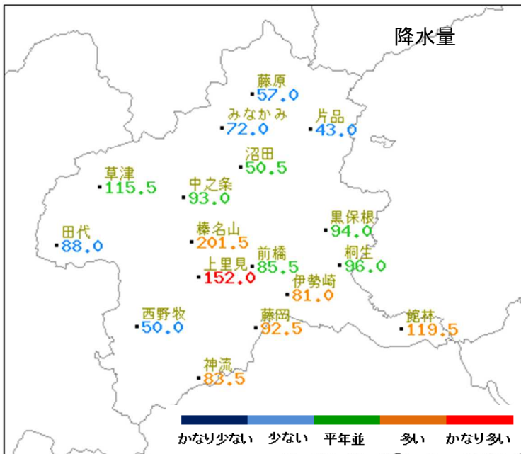
アメダス月別値 2025年4月 降水量(mm)
