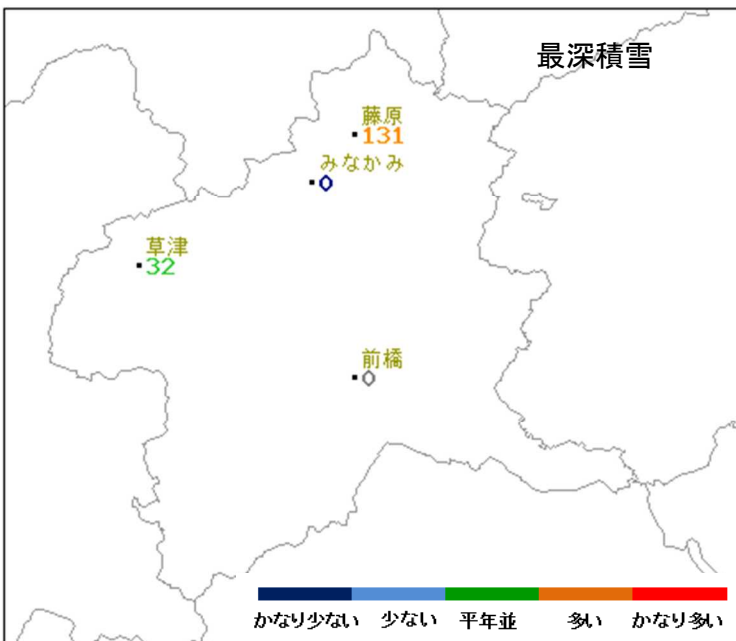
アメダス月別値 2025年4月 最深積雪(cm)
