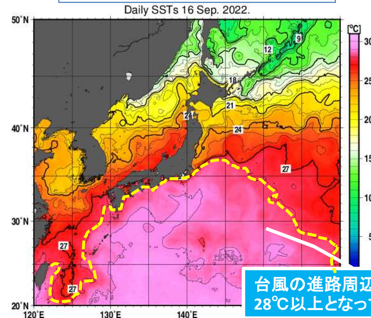
海面水温実況図 9月16日
