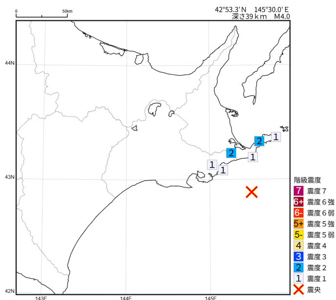
2026年 9月 9日 07時15分 釧路沖の地震の震度分布図
