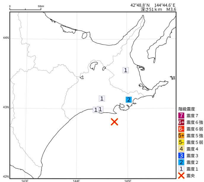
2026年 9月 4日 23時52分 釧路沖の地震の震度分布図
