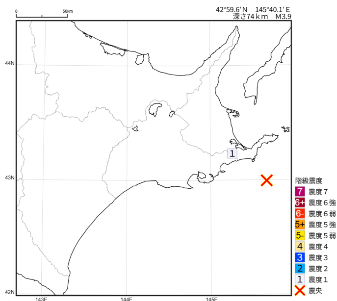
2026年 9月 8日 22時23分 根室半島南東沖の地震の震度分布図
