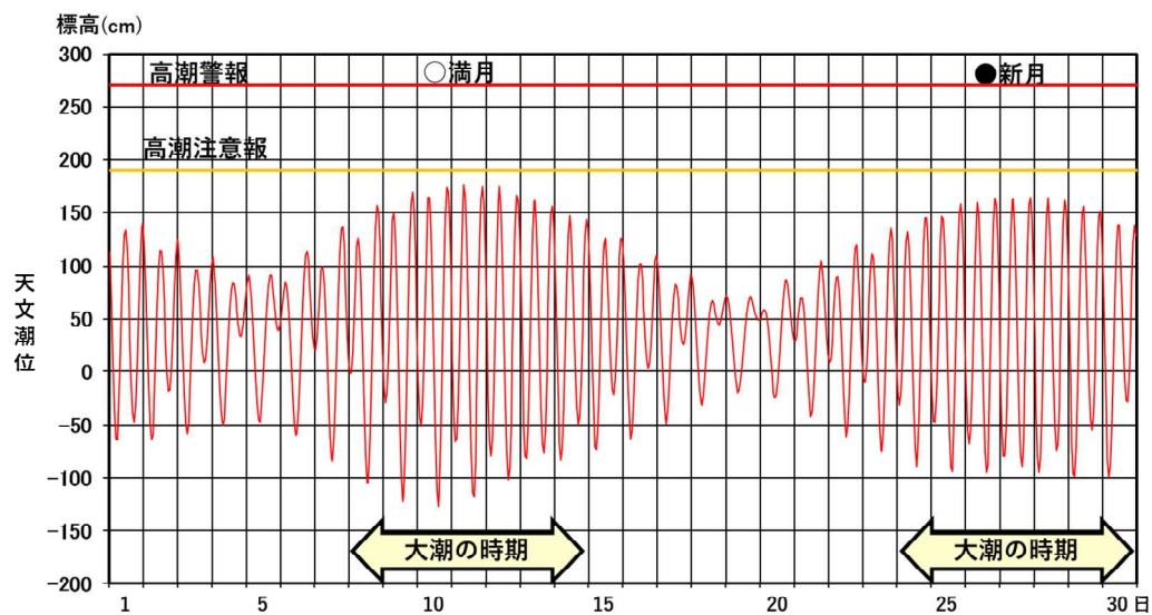
図3 苓北における2022年9月(1時間ごと)の天文潮位
