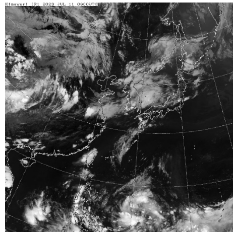
7月11日18時の地上天気図（左）と気象衛星赤外面像（右）
