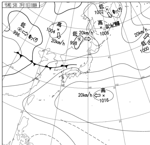
7月11日18時の地上天気図（左）と気象衛星赤外面像（右）
