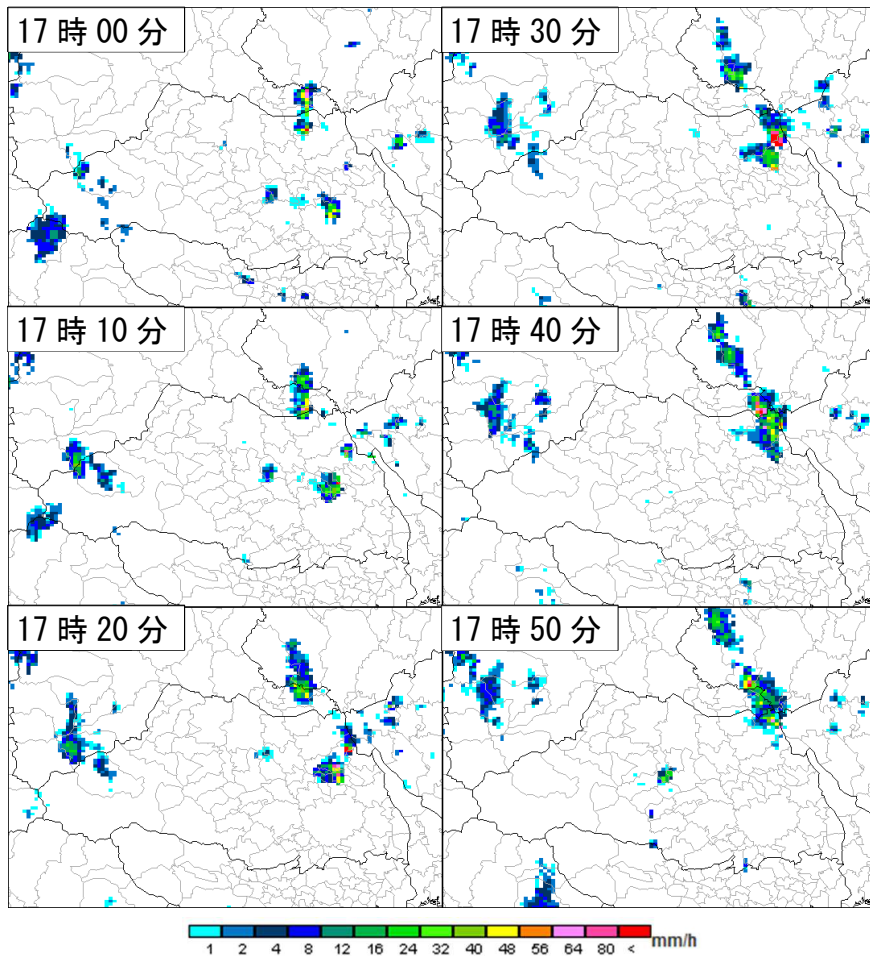
8月14日17時00分から10分毎のレーダー画像
