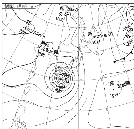
8 月 14 日 18 時の地上天気図 (左) と気象衛星赤外面像 (右)
