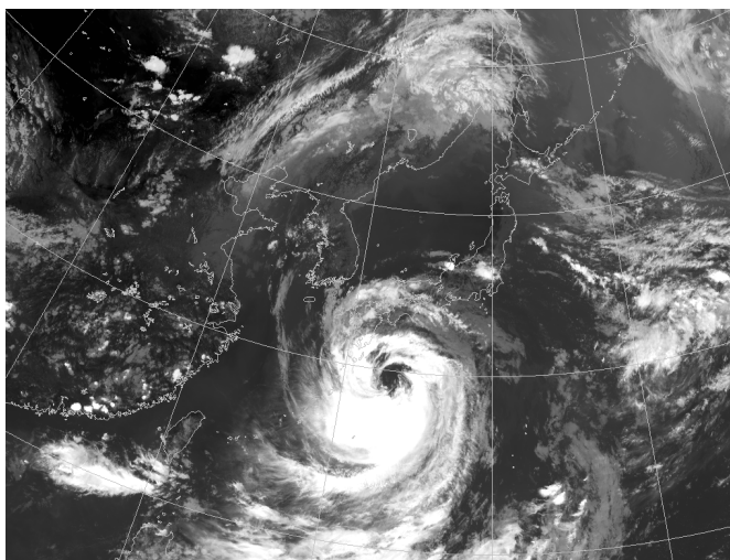
8 月 14 日 15 時の地上天気図 (左) と気象衛星赤外面像 (右)
