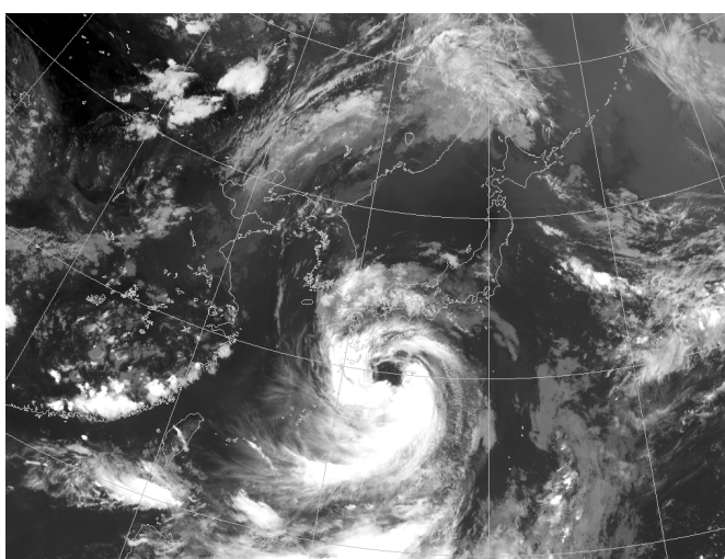
8 月 14 日 18 時の地上天気図 (左) と気象衛星赤外面像 (右)
