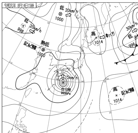
8 月 14 日 15 時の地上天気図 (左) と気象衛星赤外面像 (右)
