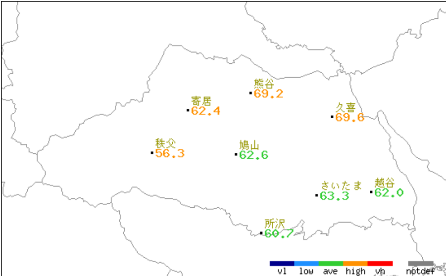
アメダス旬別値 2025年8月中旬 日照時間(h)
