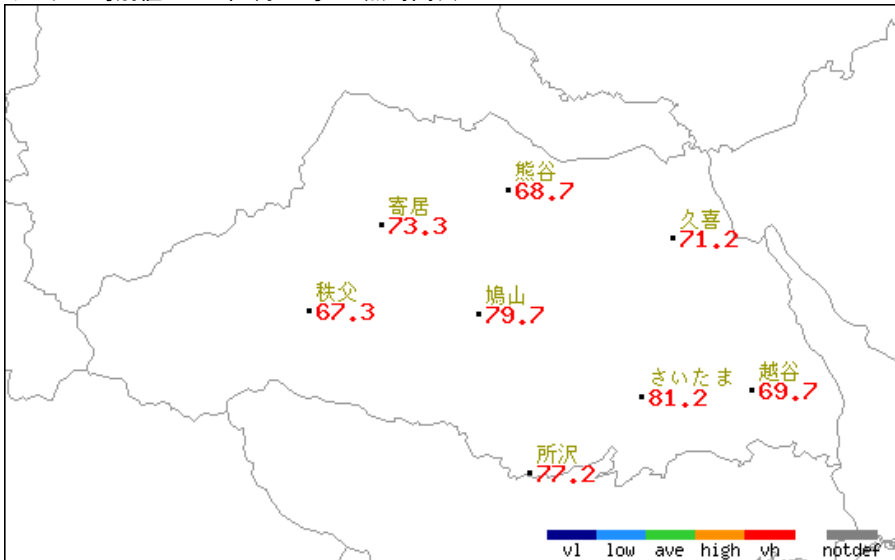
アメダス旬別値 2025年7月上旬 日照時間(h)
