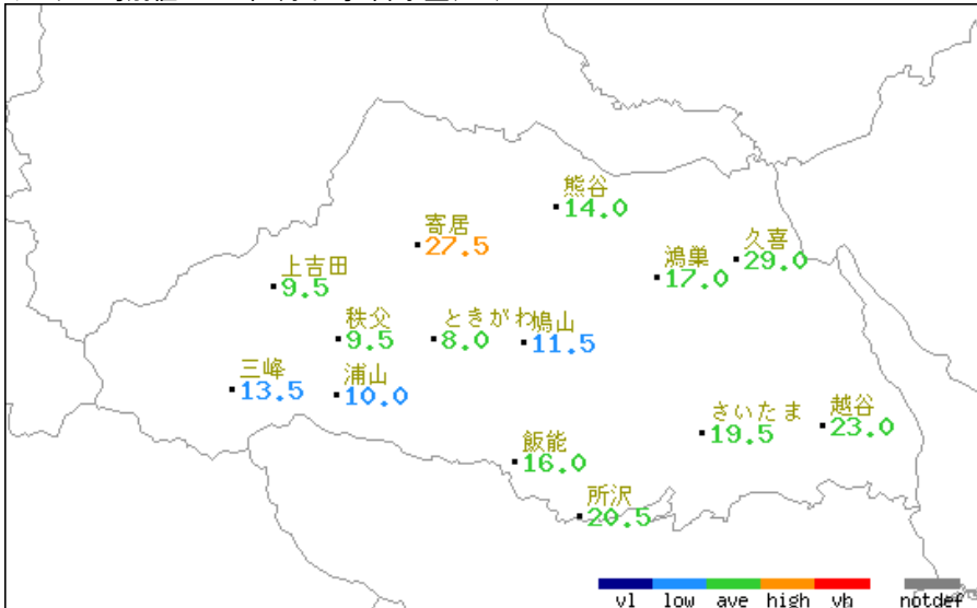
アメダス旬別値 2025年4月下旬 日照時間(h)
