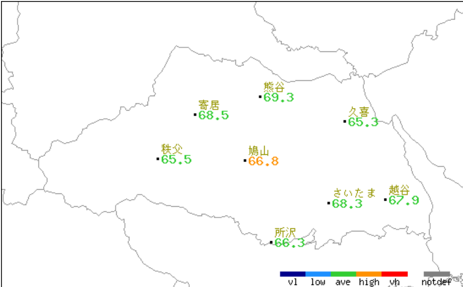
アメダス旬別値 2025年4月中旬 日照時間(h)
