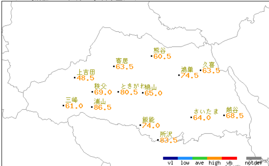
アメダス旬別値 2025年4月上旬 日照時間(h)
