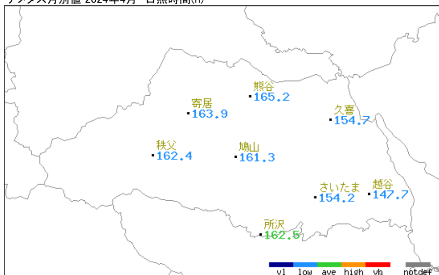
アメダス月別値 2024年4月 日照時間(h)
