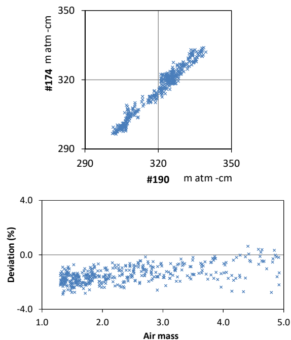
図 2 校正前の O_3 全量の比較(BR#174/BR#190)
