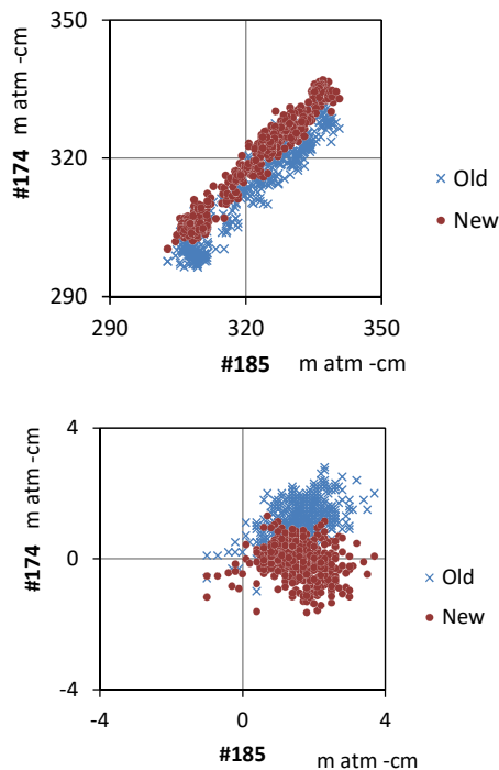
図 10 校正前後の O 3 全量の比較(BR#174/BR#185)
