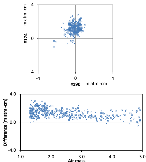
図 3 校正前の SO_2 全量の比較(BR#174/BR#190)
