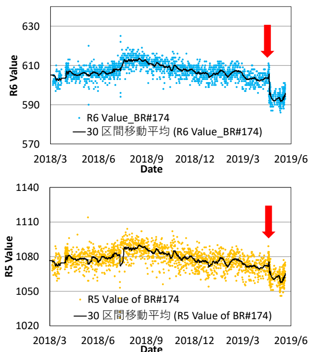
図 1 BR#174 の内部標準ランプ点検による O_3 \cdot SO_2 観測用二重比の推移(2018 年 3 月～2019 年 5 月)
